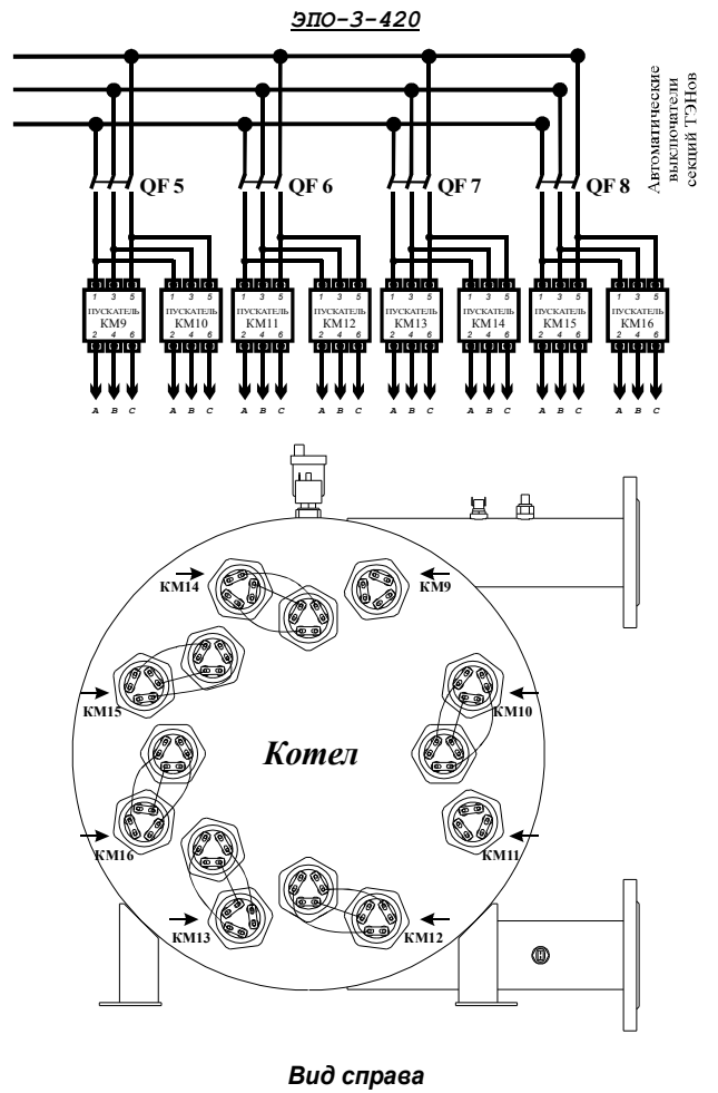
Рис. 7-2 Электрическая схема подключения
