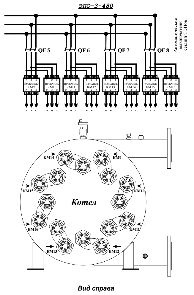
Рис. 6-2 Электрическая схема подключения
