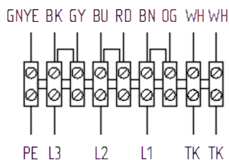
Схема №5 400В, 3ф, 50Г
