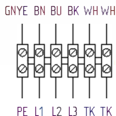
Схема №3 400В, 3ф, 50Г
