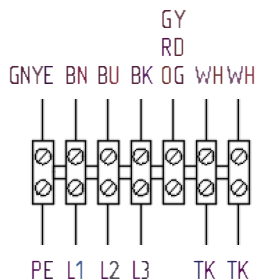
Схема №4 400В, 3ф, 50Г
