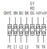
Схема №4 400В, 3ф, 50Гц
