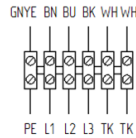
Схема №3 400В, 3ф, 50Гц
