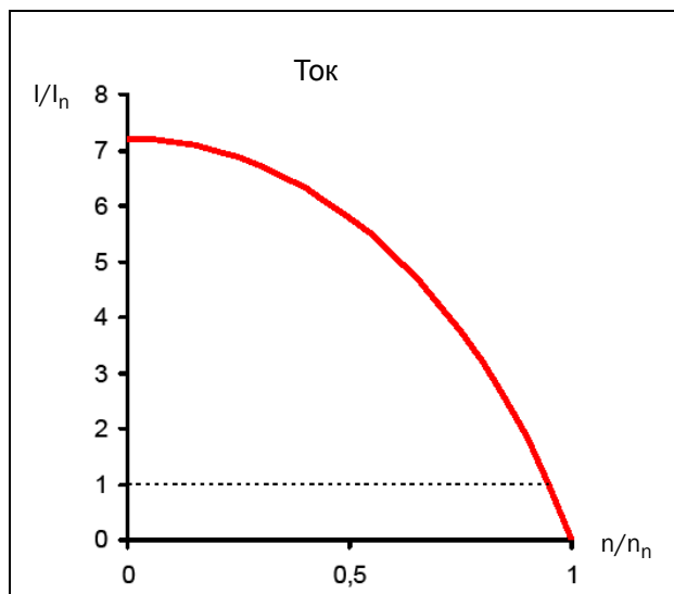
Рис. 4 Типовые характеристики тока для прямого пуска (DOL)
