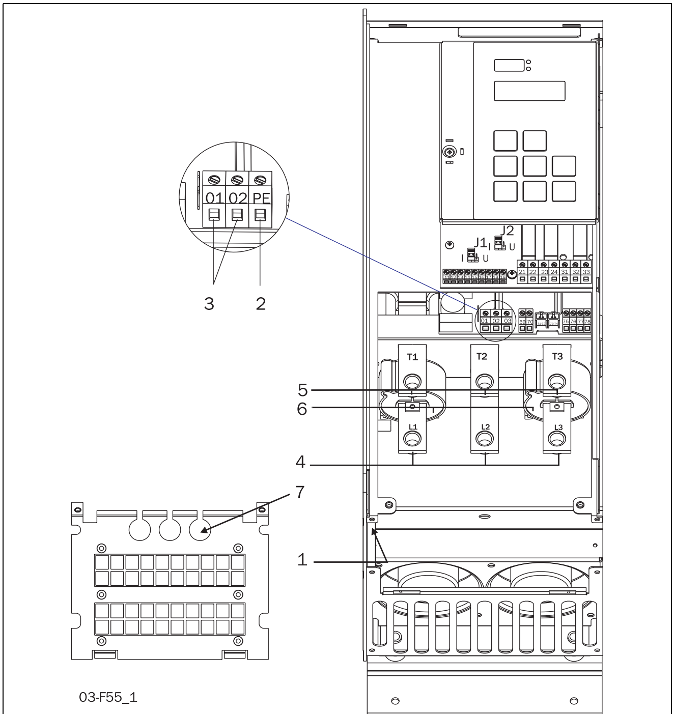
Рис. 20 Подключение MSF-110...MSF-145
