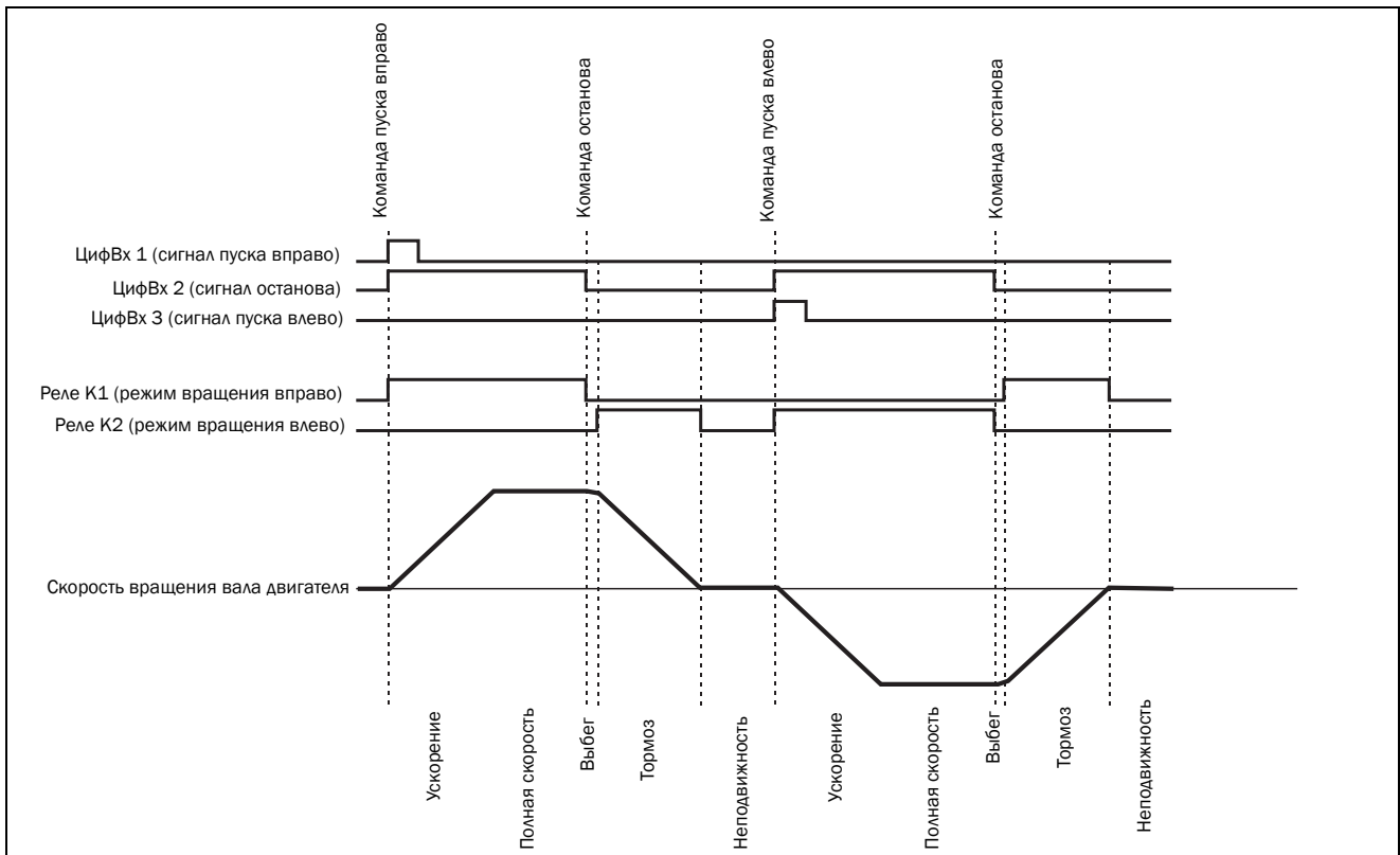
Рис. 67 Пуск право/влево с использованием торможения противотоком
