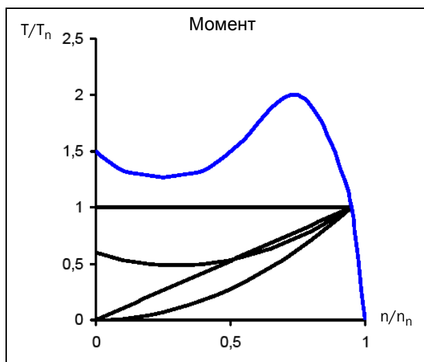
Рис. 5 Типовые характеристики момента нагрузки
