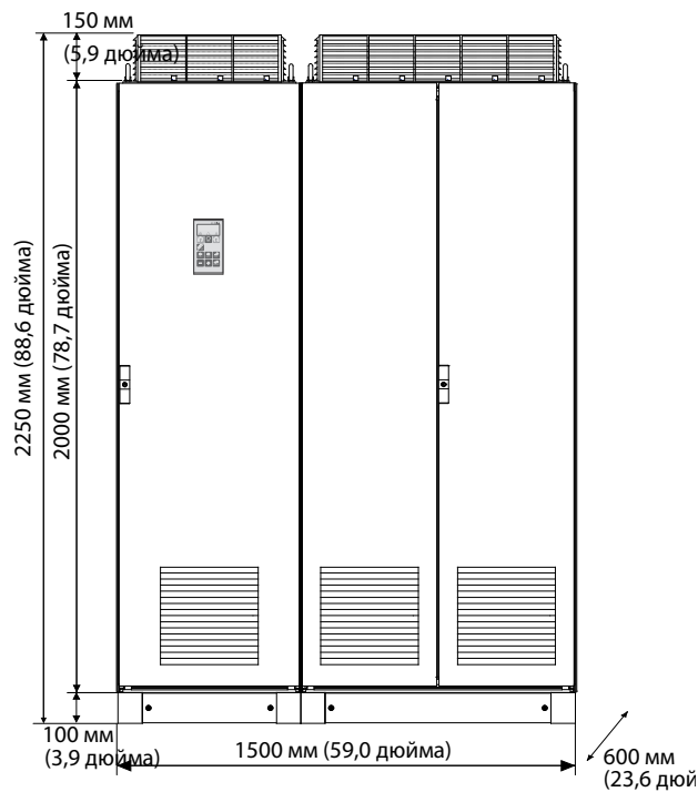
Устройство Emotron VFX48: модели от 1K15 до 1K25 (размер корпуса KA) Устройство Emotron VFX69: модели 905–995 (размер корпуса KA69)
