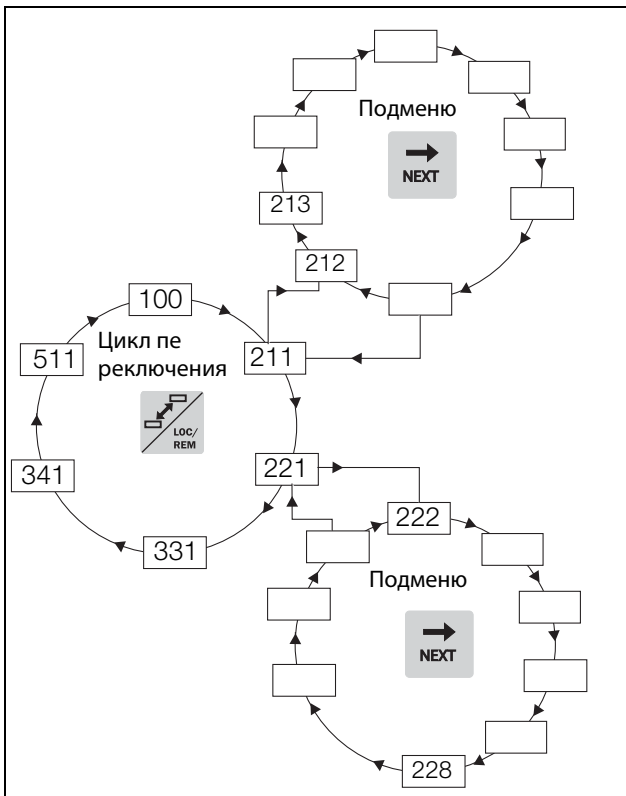
Рис. 89 Пример цикла переключения.
