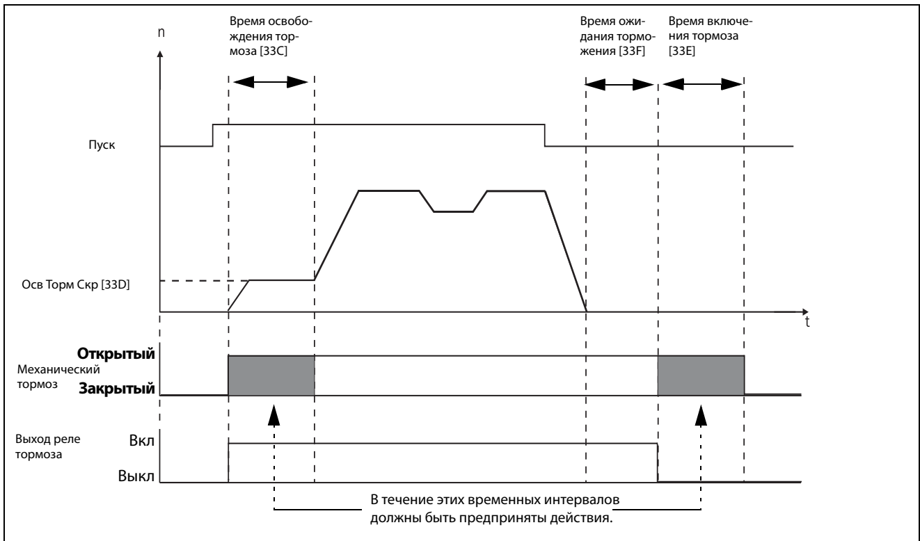
Рис. 103 Функции торможения
