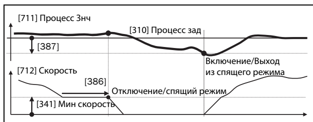
Рис. 112 Отключение/спящий режим ПИД при обычном ПИД-управлении
