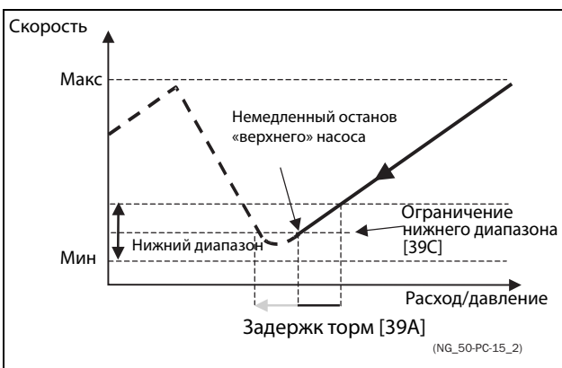
Рис. 118 Ограничение нижнего диапазона
