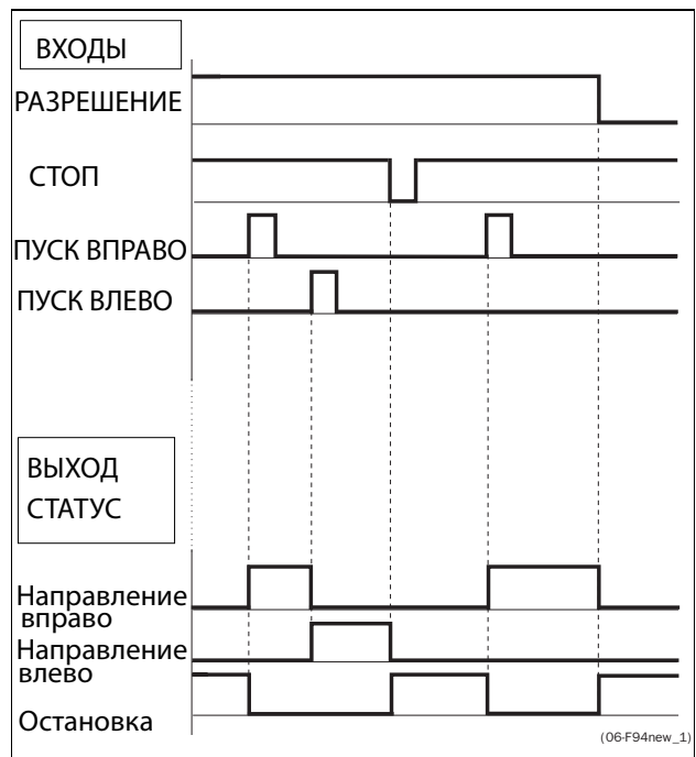
Рис. 74 Состояние входов и выходов при управлении фронтом
