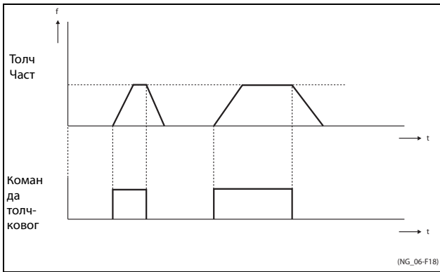
Рис. 107 Команда толчкового режима
