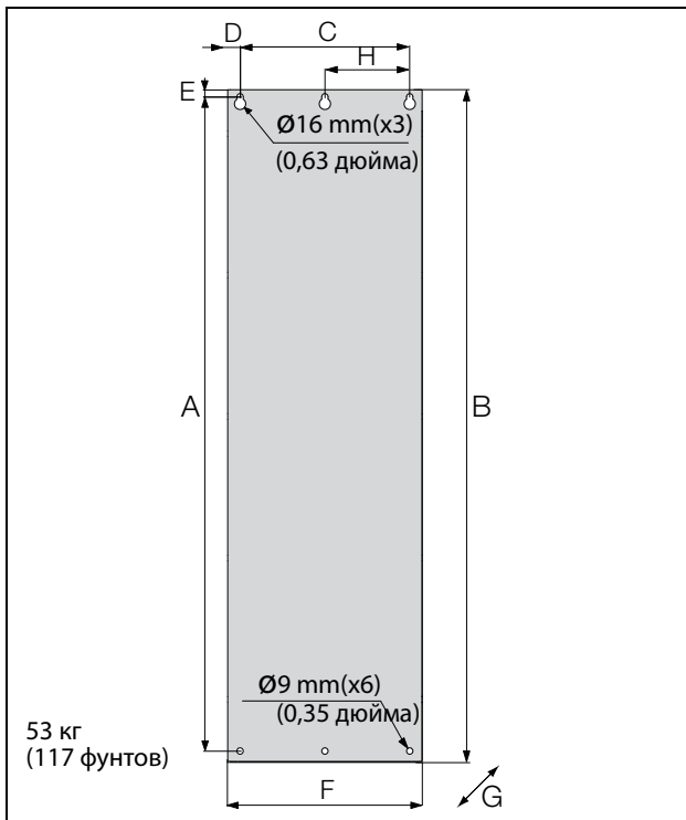
Рис. 22 Устройство VFX/ моделей от 48-142 до 48-171 (размер корпуса E2).
