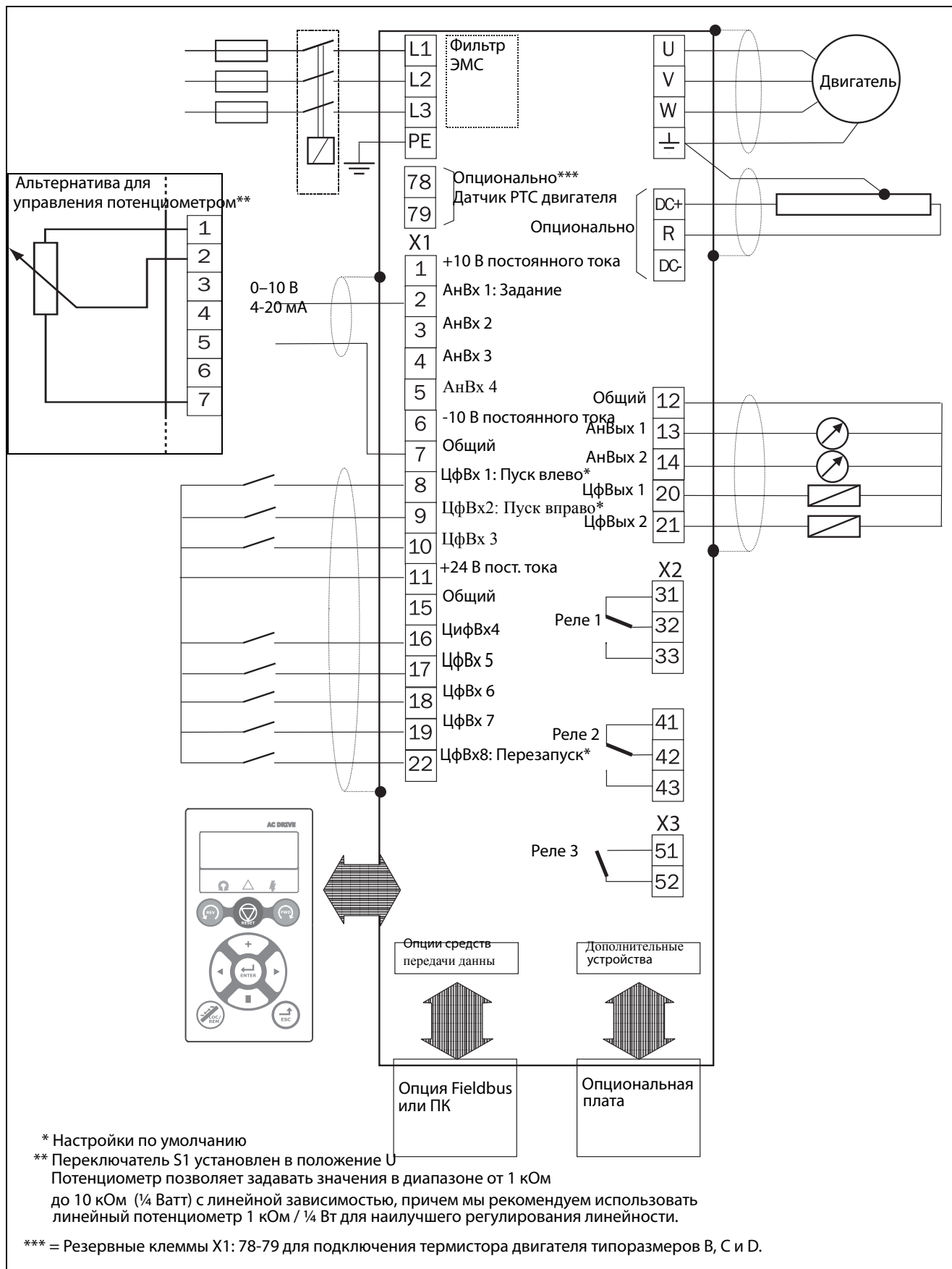
Рис. 57 Пример подключения
