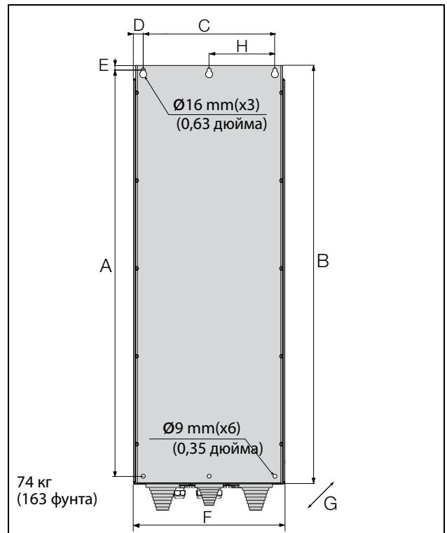
Рис. 20 Устройство Emotron VFX моделей с 48-210 по 295 (размер корпуса F), Устройство Emotron VFX моделей с 69-82 по 200 (размер корпуса F69).
