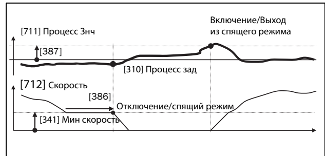
Рис. 113 Отключение/спящий режим ПИД при инвертированном ПИД-управлении
