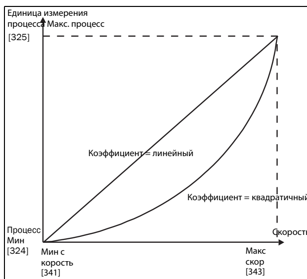
Рис. 96 Коэффициент
