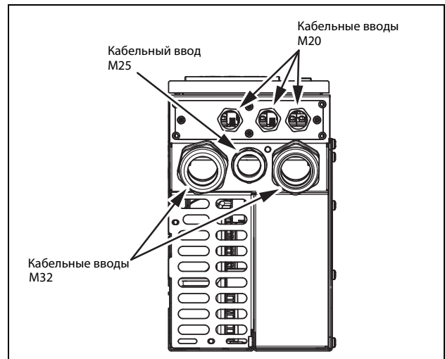
Рис. 13 Кабельный интерфейс для подключения электрической сети, электродвигателя и управления, устройство Emotron VFX моделей 69-002–025 (размер корпуса С69).
