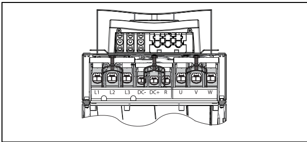
Рис. 23 Вид снизу, устройство Emotron VFX/ моделей от 48-142 до 48-293 (размер корпуса E2 и F2) с кабельным интерфейсом для подключения электрической сети, электродвигателя, опции DC+/DC-, тормозного резистора и управления (принципиальная схема).
