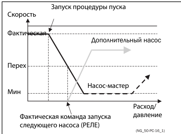
Рис. 119 Скорость перехода
