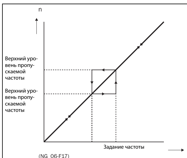
Рис. 106 Пропускаемая частота
