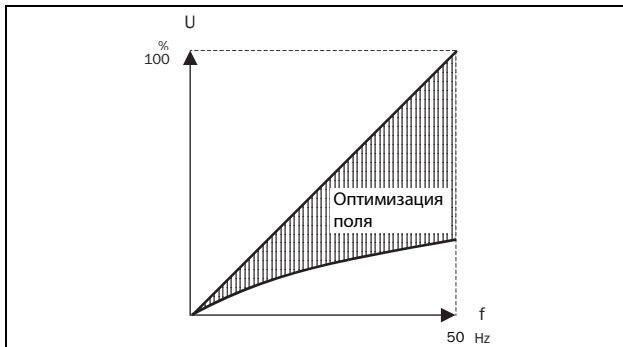
Рис. 109 Оптимизация поля
