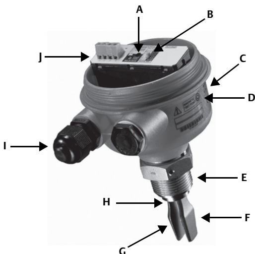
Рисунок 1. Функции Rosemount 2120
