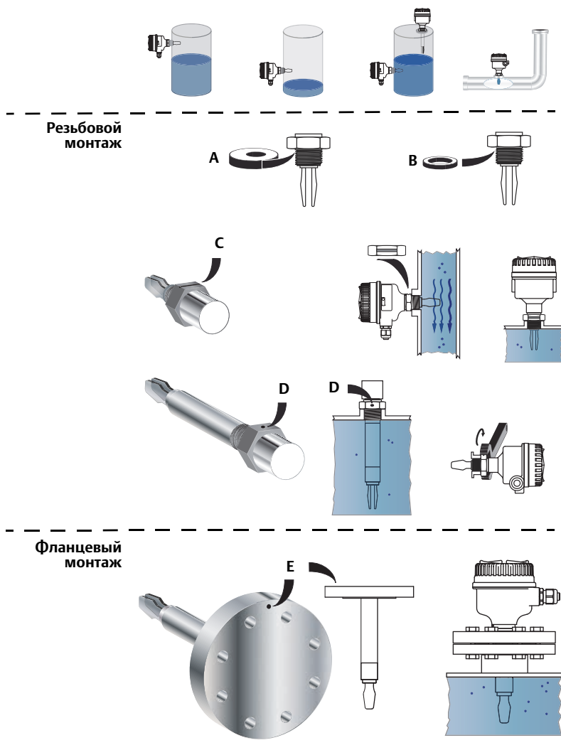
Рисунок 5. Пример установки
