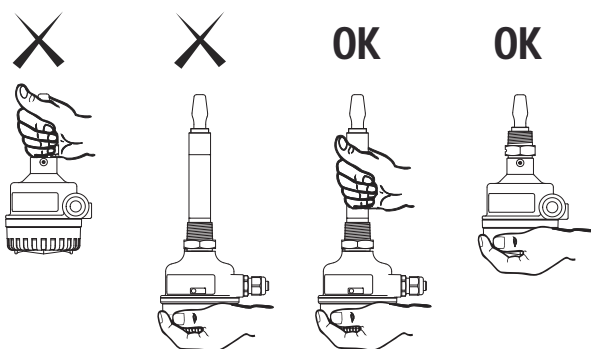
Рисунок 2. Переноска Rosemount 2120
