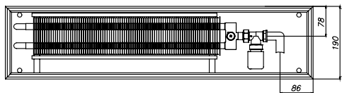
EKN.190.150, вид сбоку
