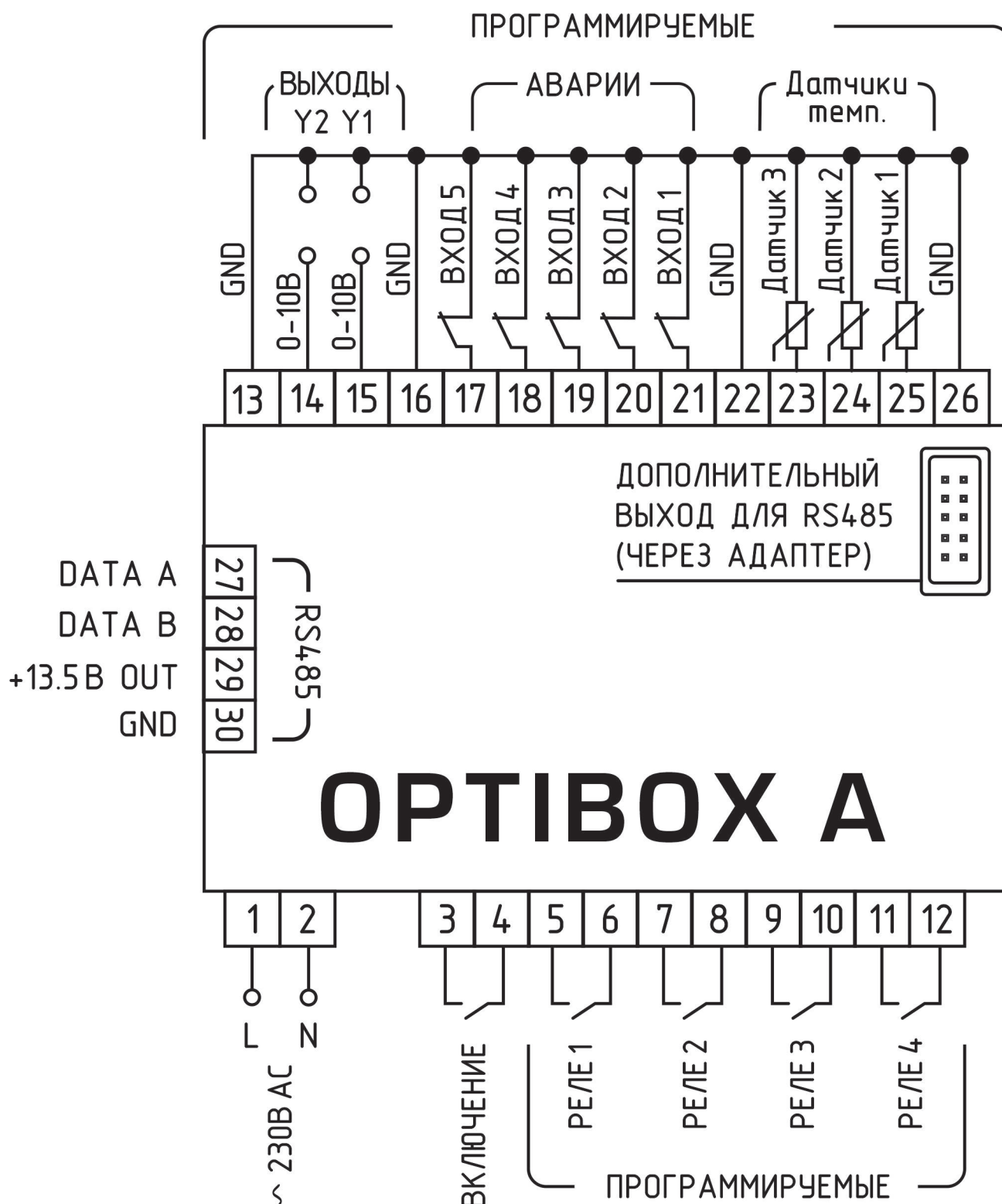
Рис. 2.1 Назначение клемм контроллера.
