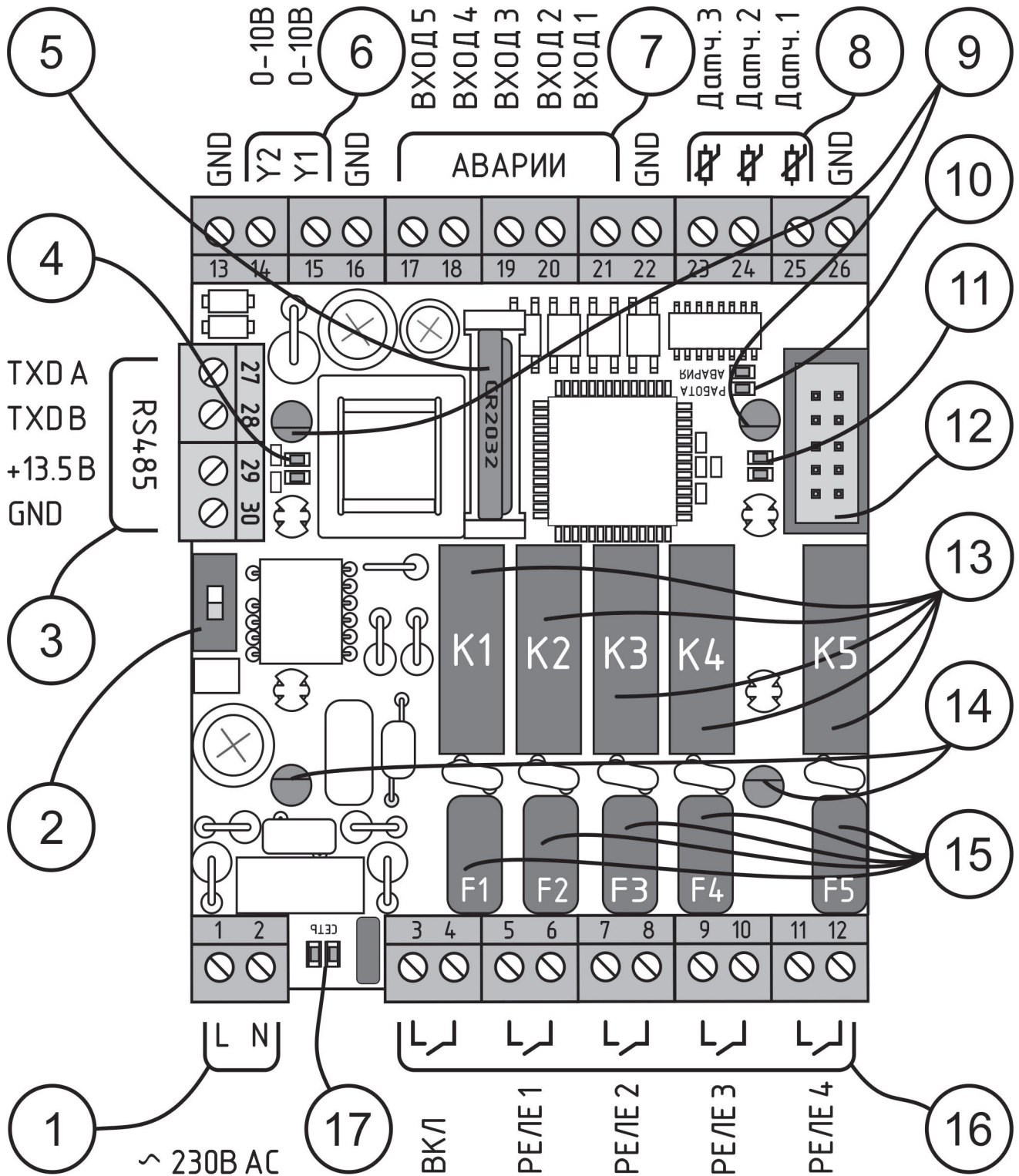
Рис. 1.1. Основные элементы и элементы индикации контроллера
