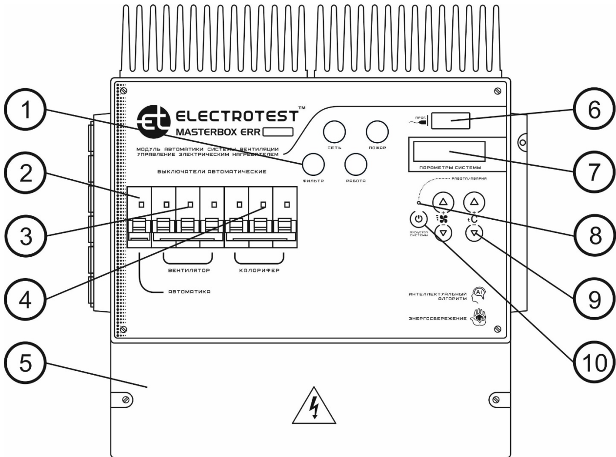
Рис. 1. Функциональные элементы модуля.
