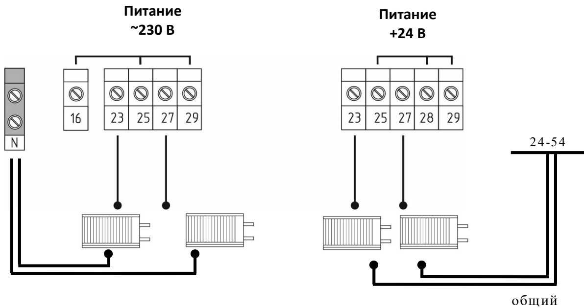
Рис. 8.2. Подключение двухконтурного фреонового охладителя с собственной автоматикой.
