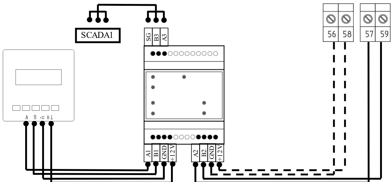
Рис. 13. Подключение к SCADA-системе.
