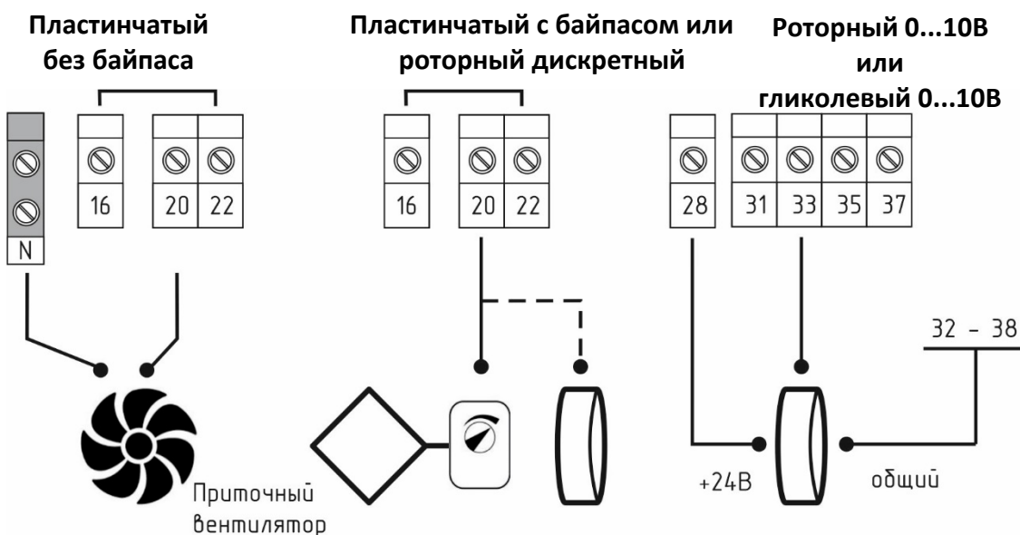
Рис. 4. Подключение рекуператора.
