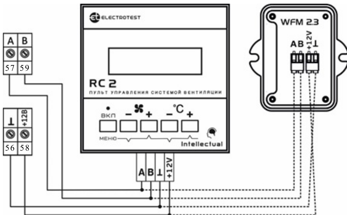
Рис. 12. Подключение пульта дистанционного управления и модуля Wi-Fi
