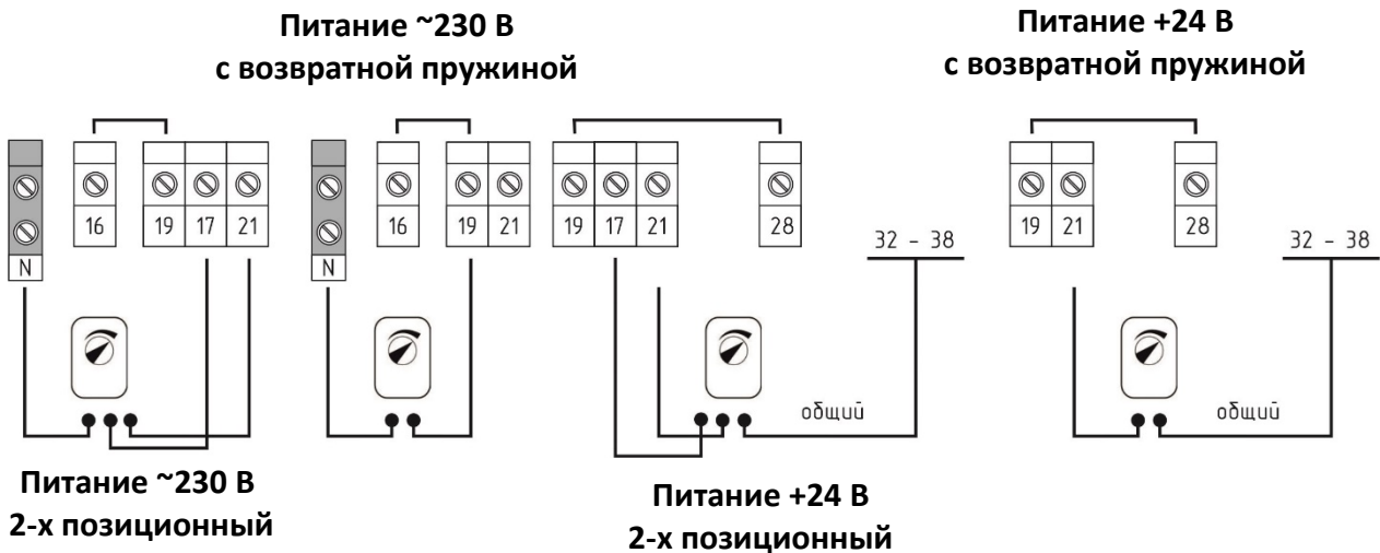
Рис. 5. Подключение привода заслонки наружного воздуха.
