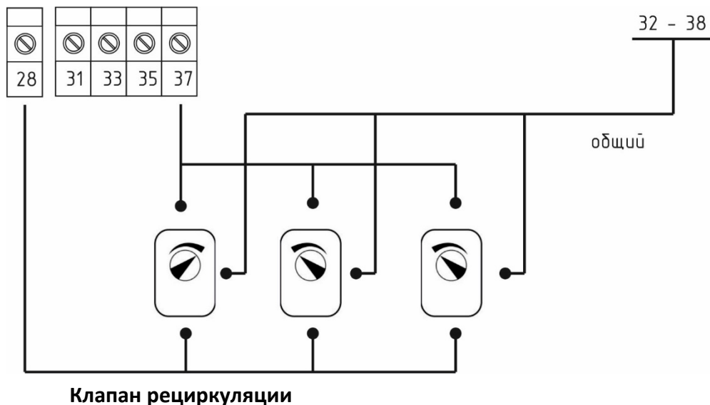
Рис. 10. Подключение заслонок рециркуляции
