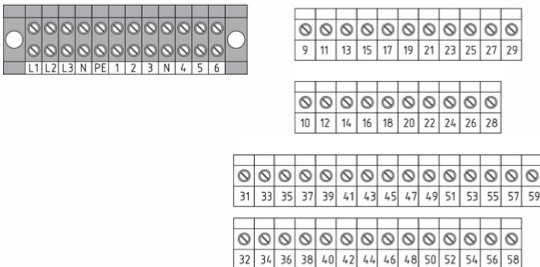
Рис. 2. Назначение клемм модуля.
