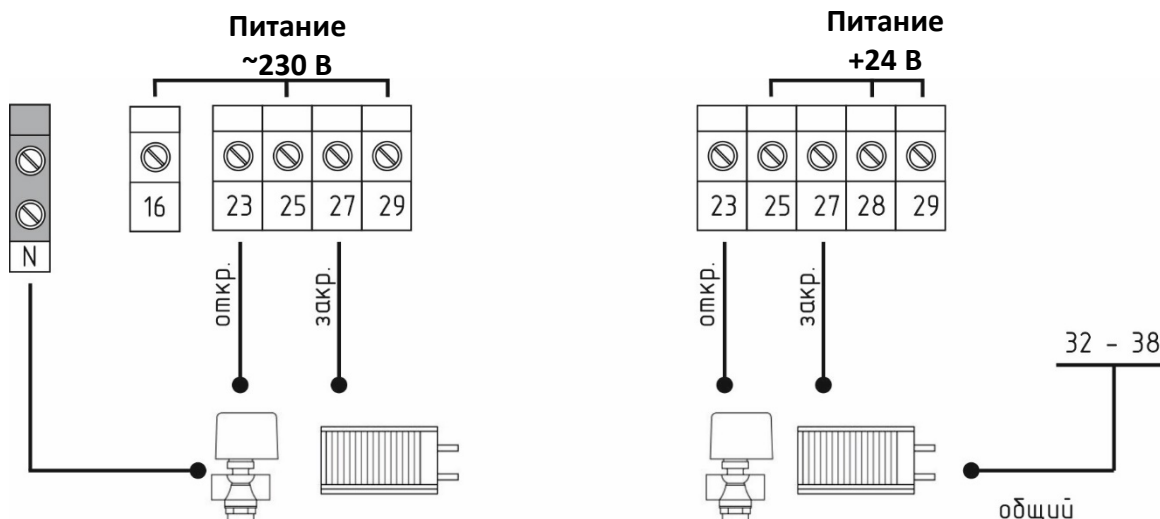
Рис. 8.1. Подключение одноконтурного фреонового охладителя без автоматики.
