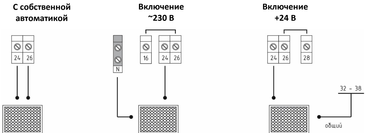
Рис. 9. Подключение увлажнителя
