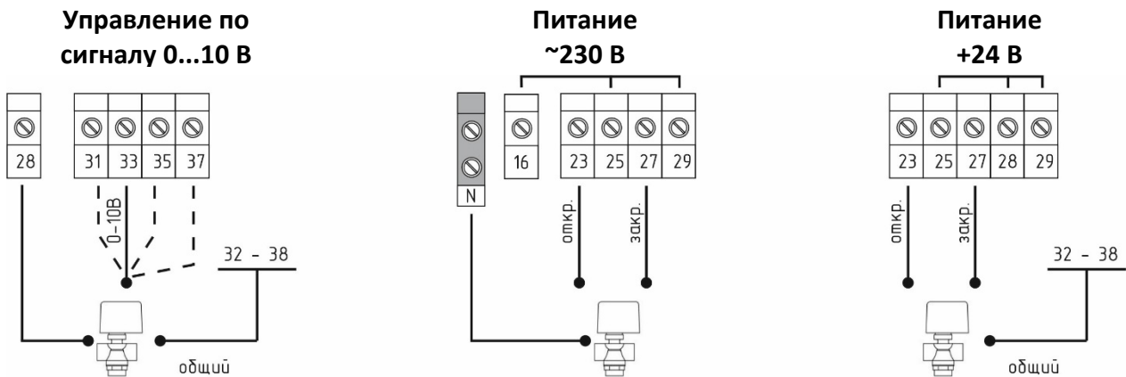
Рис. 7. Подключение привода клапана холодной воды
