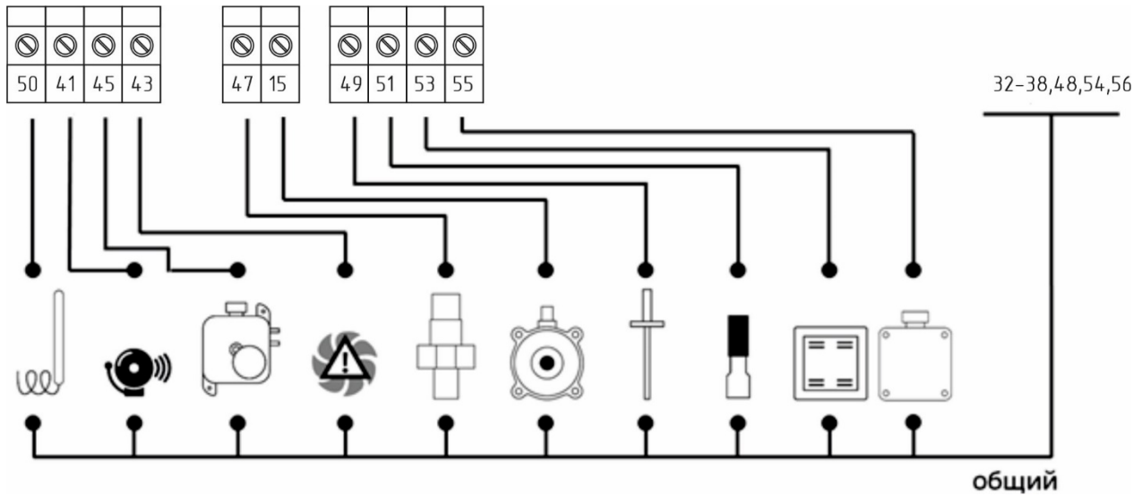
Рис. 11. Подключение датчиков.
