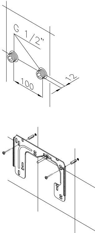
рис. 3 Установка прибора
