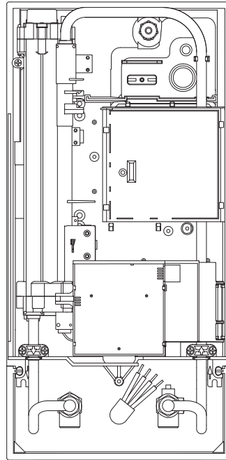
рис. 3 Установка прибора
