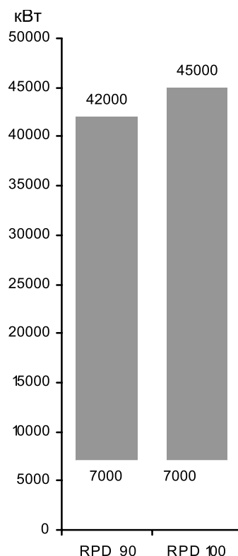
Диапазон мощности
