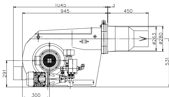
Размерный эскиз EK 6.240 / 300 L-EUF
