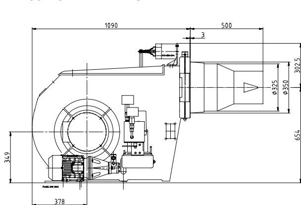
Размерный эскиз EK 7... L-RUF
