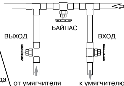
Байпасный вентиль
