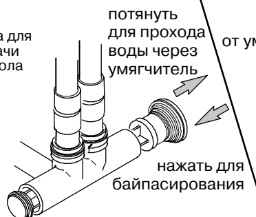
Байпасный вентиль
