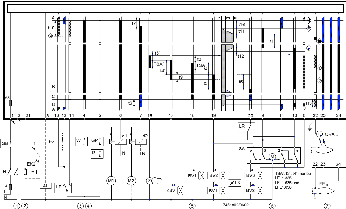
Схема подключения
