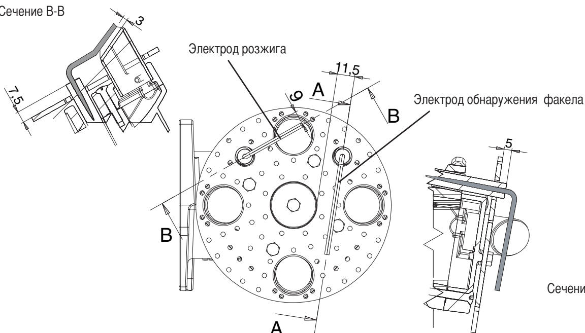
Сечение В-В
