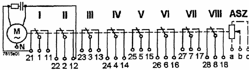
Соединительные клеммы
