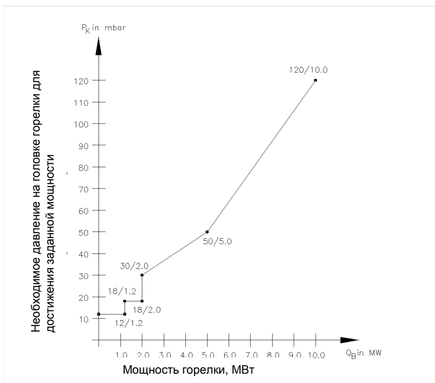
Рис. 2 Необходимое давление на головке горелки в зависимости от мощности горелки
