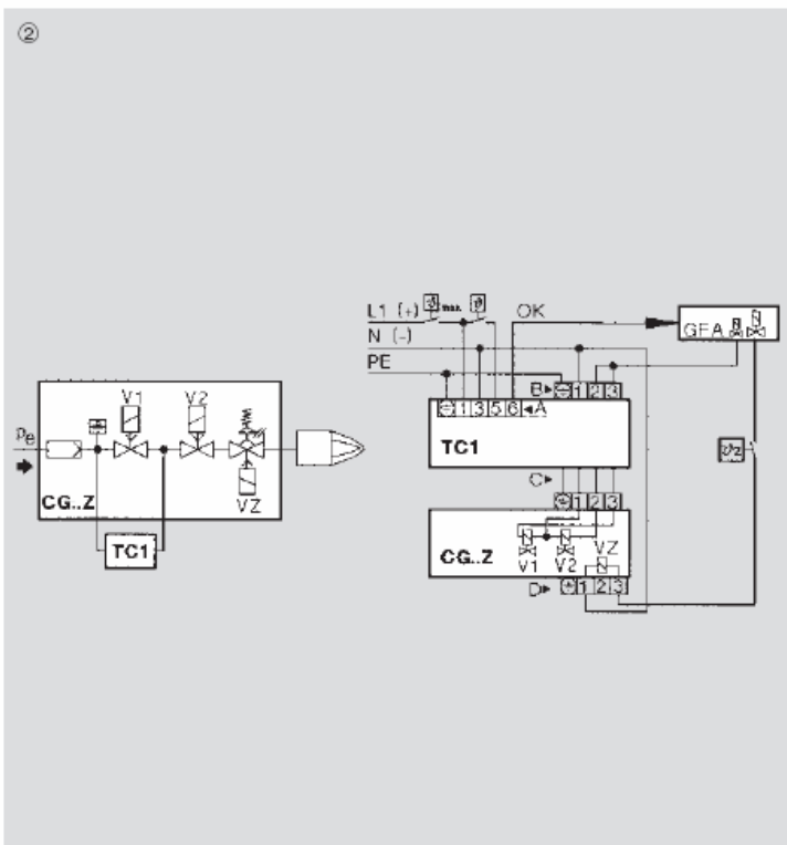
GFA Gasfeuerungsautomat / burner control unit/ автомат управления горелками
