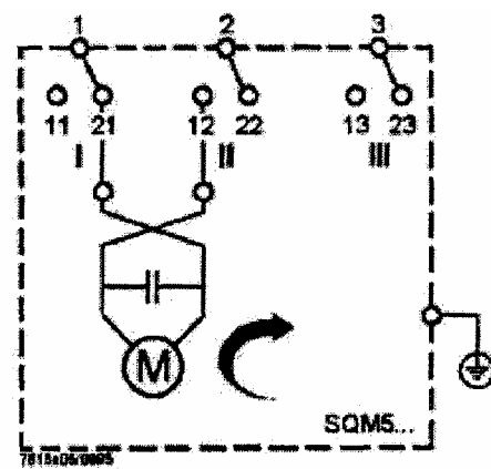
Правое вращение
