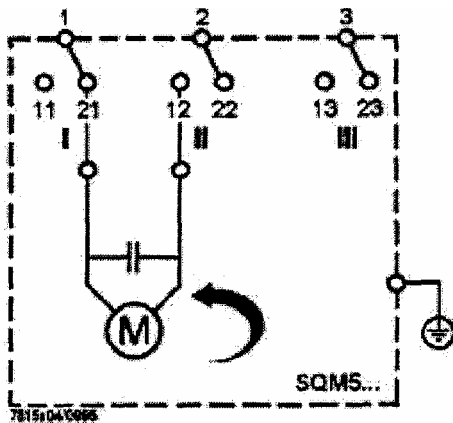
Левое вращение
