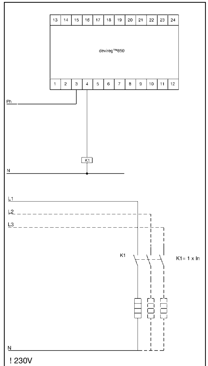
Рис. D. Кровля, 1-3 фазы, 1-3 кабеля на 230
