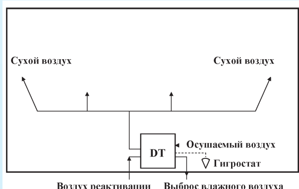
Установка осушителя на складе
