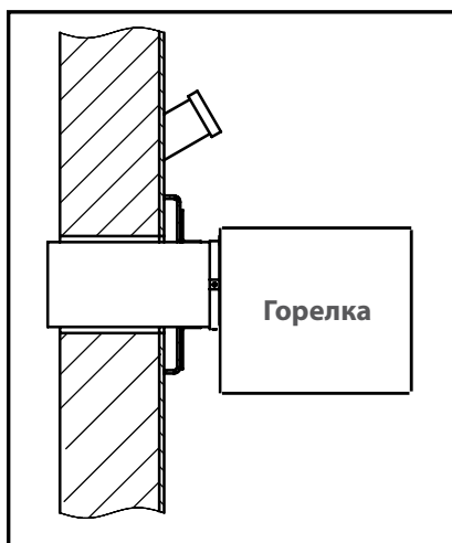
Рис. 2 Требования к установке в котел горелки DanVex.
