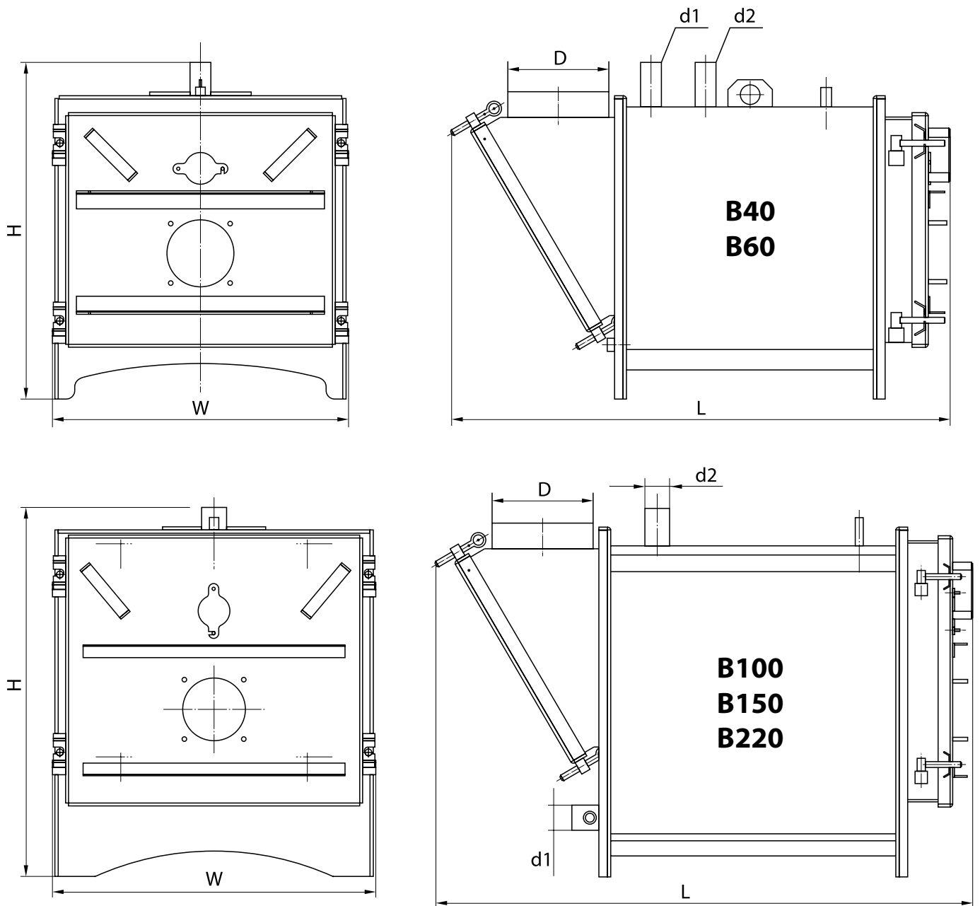
Рис. 3 Габариты котлов
