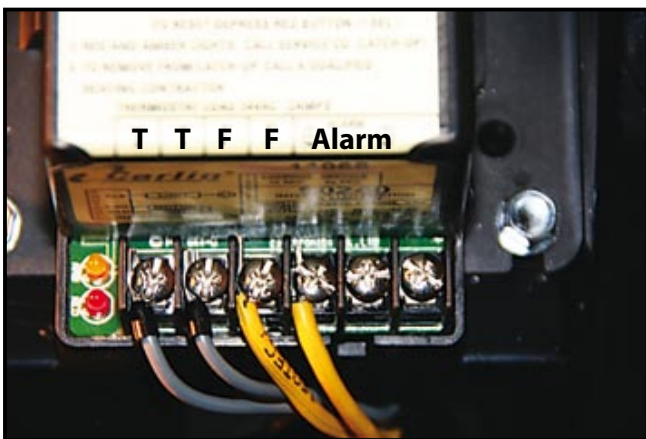
Контролер горелки
