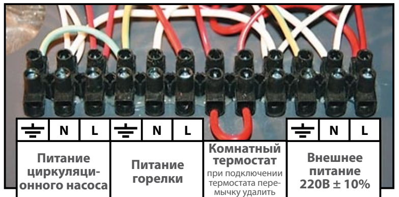
Клеммная колодка в пульте управления котлом
