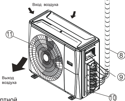
Наружный блок
