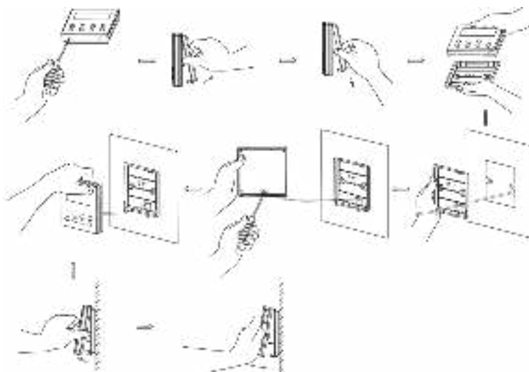
Рис.27 Монтаж проводного пульта управления
