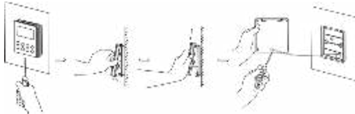
Рис.28 Демонтаж проводного пульта управления
