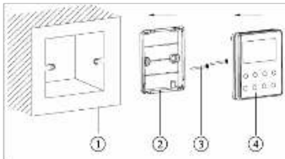
Рис. 26: Стандартные части проводного пульта управления
