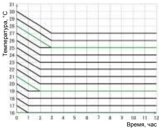
Рис.15 График изменения температуры в режиме «HEAT» («ОБОГРЕВ») с включенной функцией «Сон»
