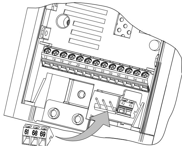
Рисунок 3.6 Расположение клемм управления
