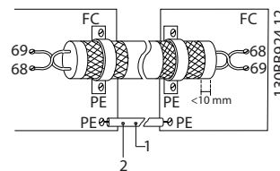
Рисунок 3.10 Кабели из витой пары без клеммы 61
