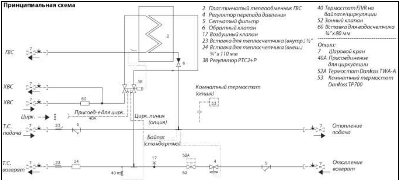
Рис. 13. Принципиальная схема МТП модификации Akva Lux II TDP-F с теплоизоляцией
