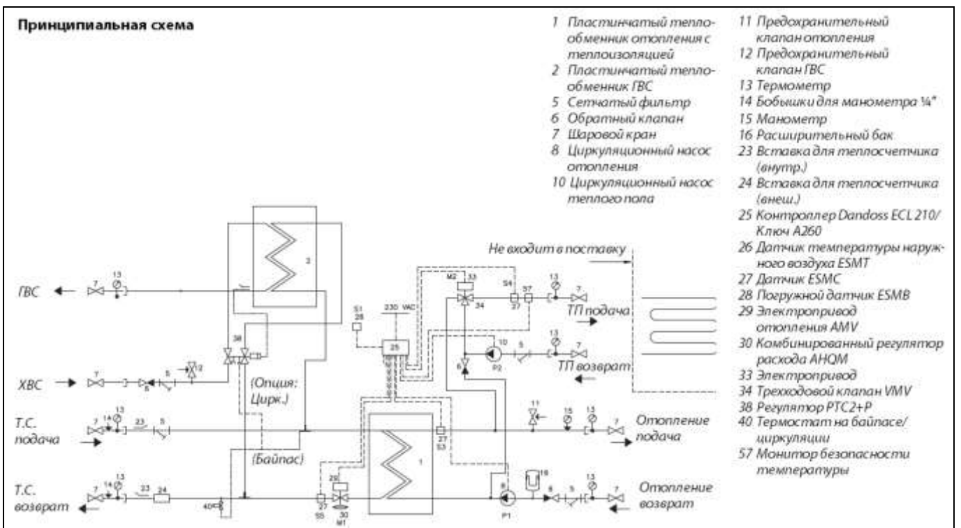
Рис. 20. Принципиальная схема МТП модификации Aqua Lux II VX H2WP, ECL, 2 HE
