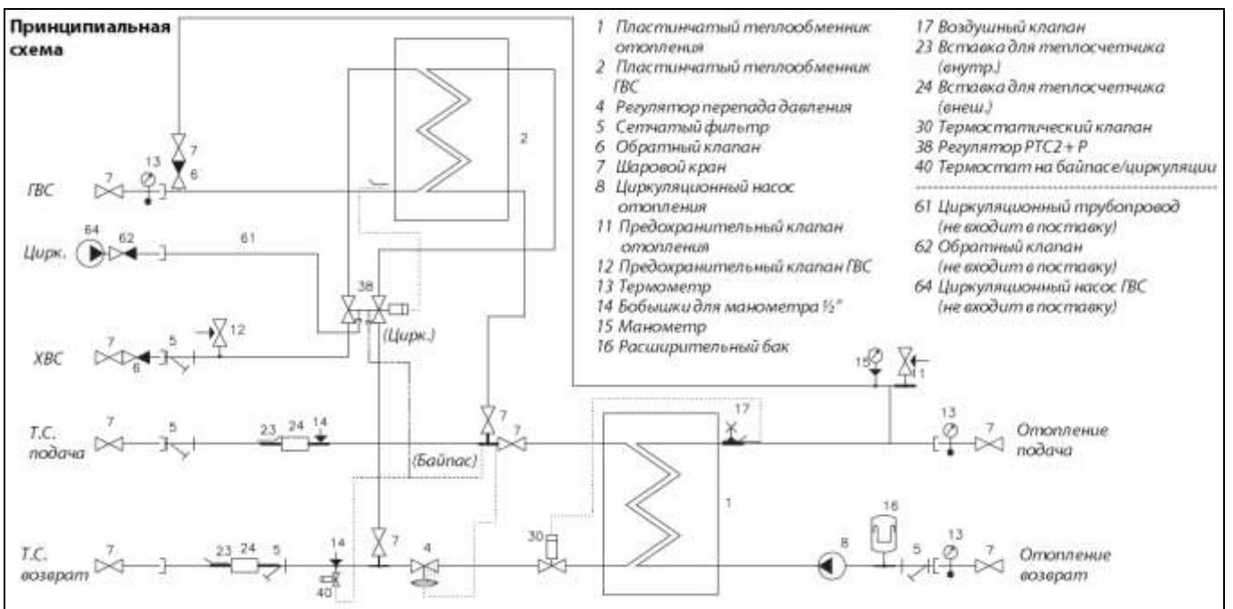
Рис. 18. Принципиальная схема МТП модификации Aqua Lux II VX
