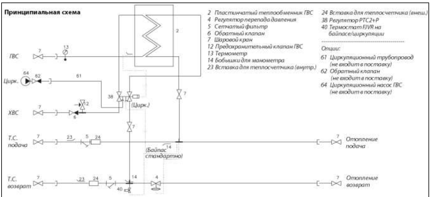
Рис. 16. Принципиальная схема МТП модификации Aqua Lux II TD с теплоизоляцией
