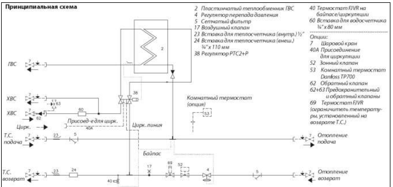
Рис. 14. Принципиальная схема МТП модификации Akva Lux II TDP-F
