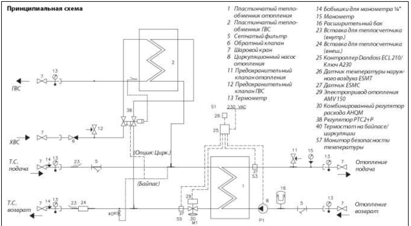
Рис. 19. Принципиальная схема МТП модификации Aqua Lux II VX HWP, ECL, 1 HE
