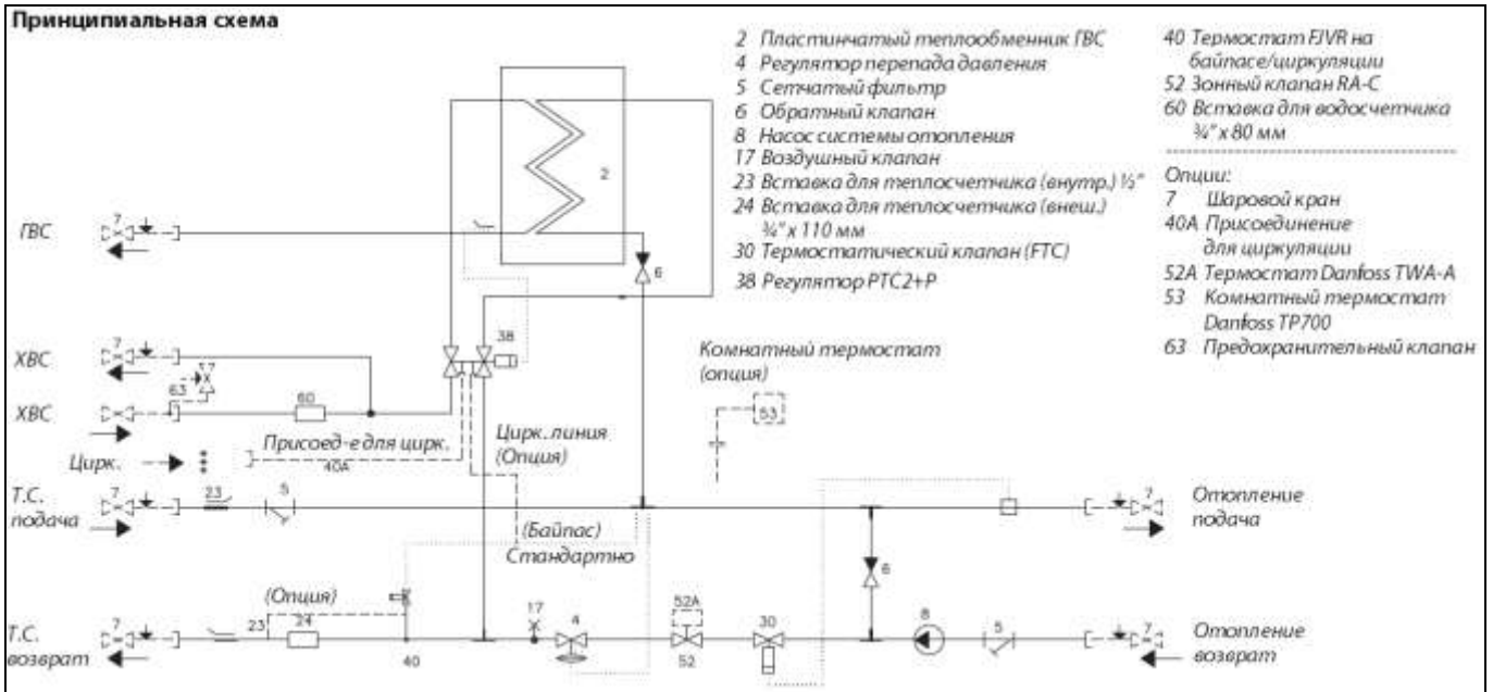
Рис. 15. Принципиальная схема МТП модификации Aqua Lux II S-F
