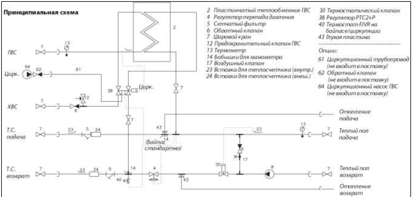
Рис. 17. Принципиальная схема МТП модификации Aqua Lux II S с теплоизоляцией
