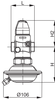
AVPB-F (PN16) DN 15 - 32
