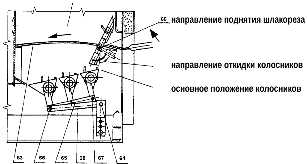
Рис.5 Отдельные части котла DOR – 12
