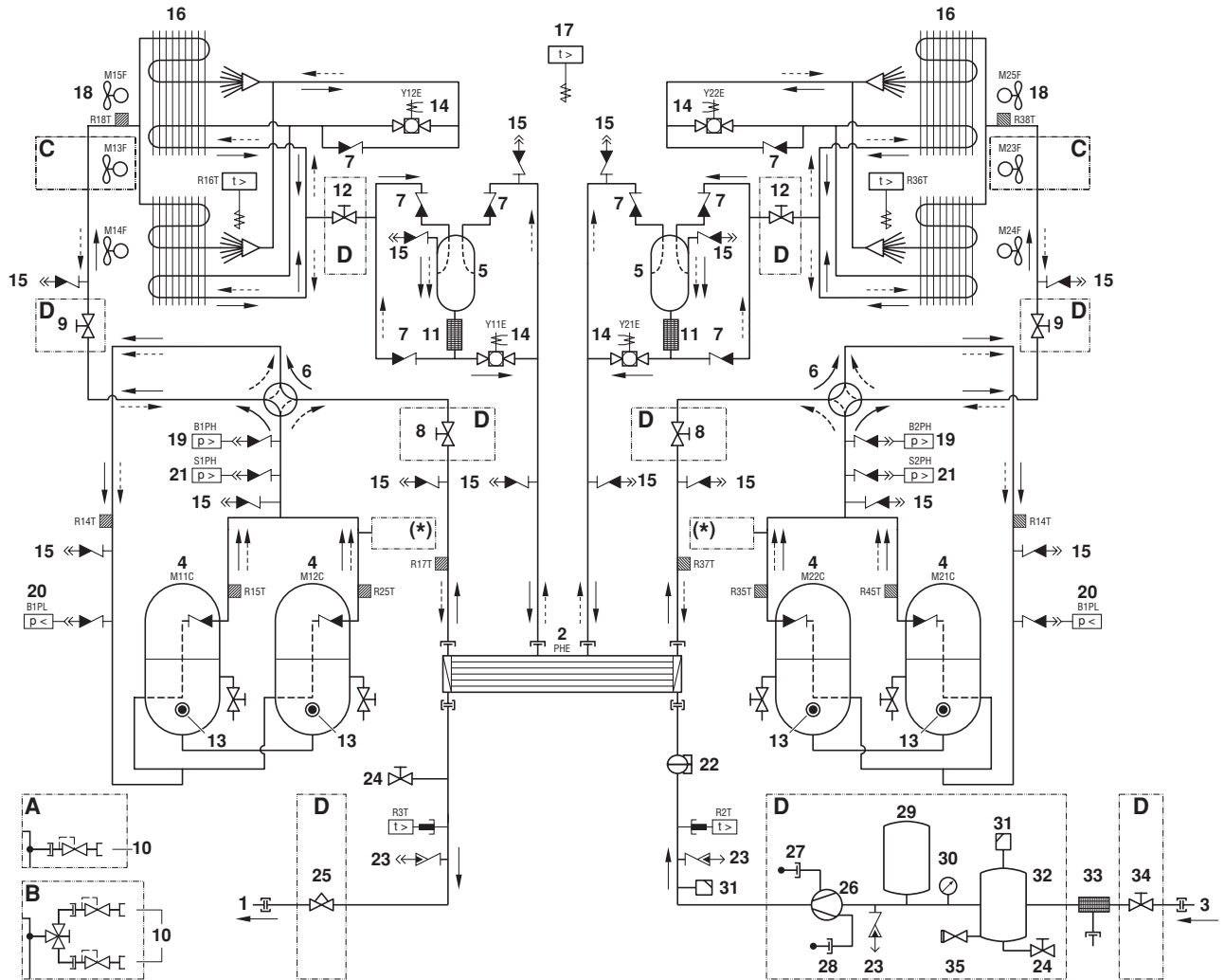
Рисунок - Функциональная схема
