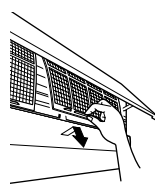
Фотокаталитический титан-апатитовый фильтр очистки воздуха Воздушный фильтр Каркас фильтра Выступ
