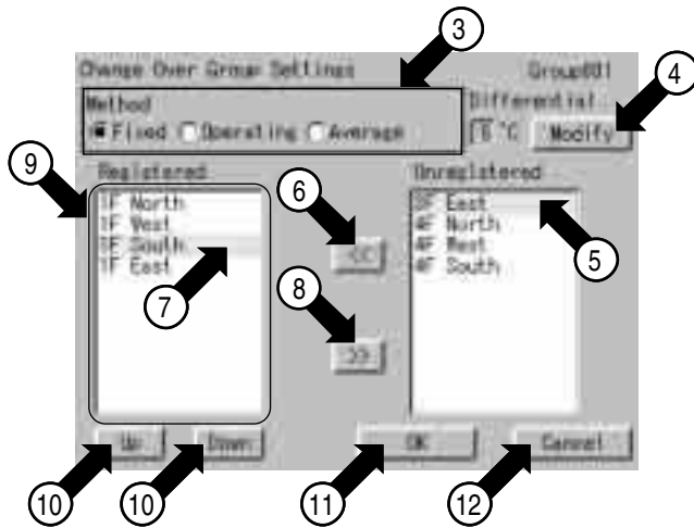
Экран 2 Установки группы автоматического переключения охлаждение / обогрев
