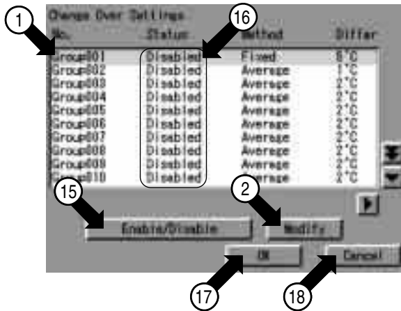
Экран 1 Установки переключения
