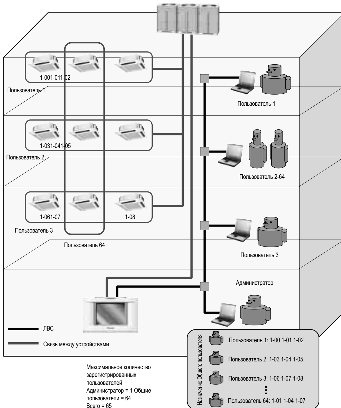
Рисунок 1: Пример установки пользователя
