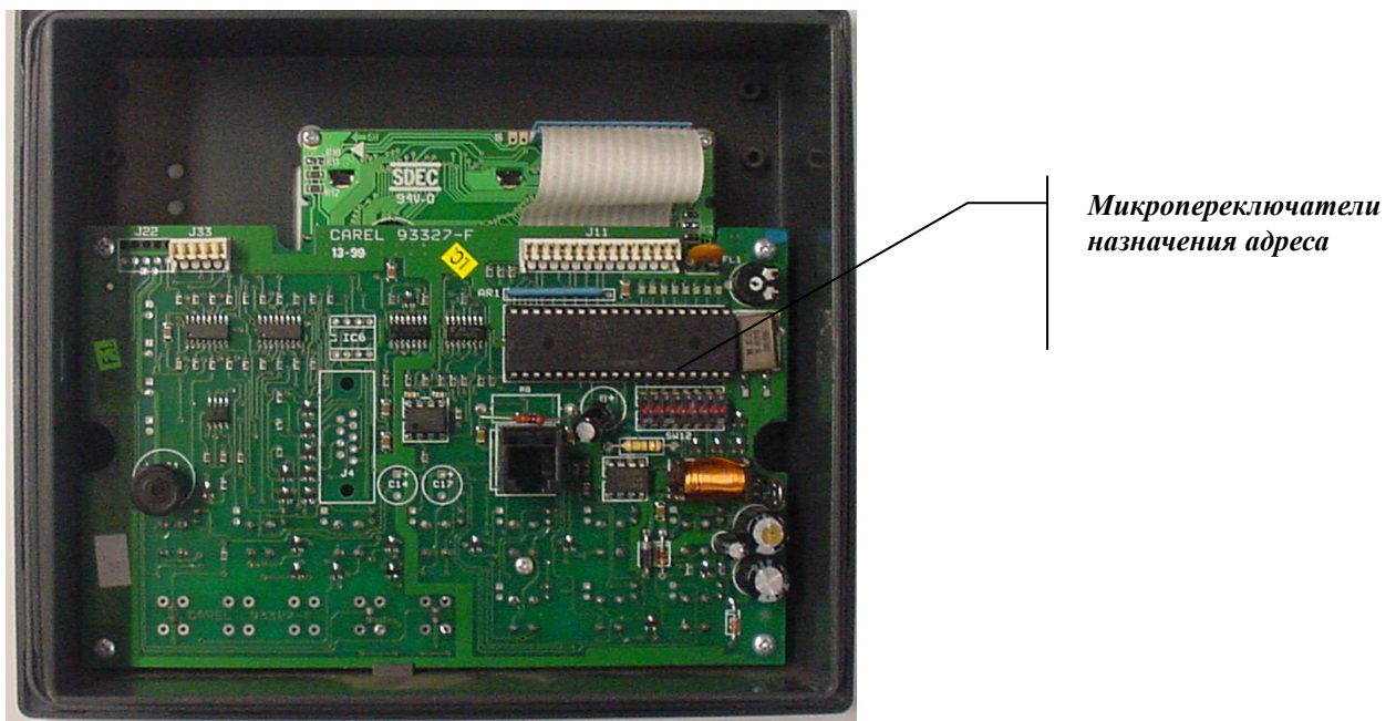
Рис. 2 – Панель управления – вид сзади
