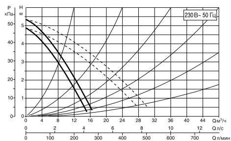
ДМН 60/280.50 Т
