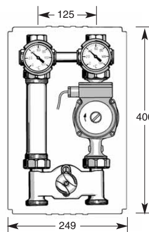
Насосный модуль M4 (Со смесительным клапаном)
