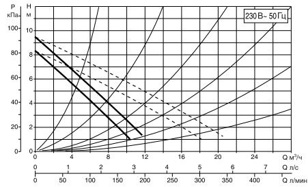
ДМН 30/280.50 Т
