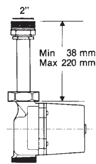
Удлинитель с резьбой 2"
