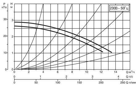
ВМН 60/280.50 Т
