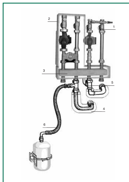
Многоконтурная система модулей, соединенных при помощи коллектора
