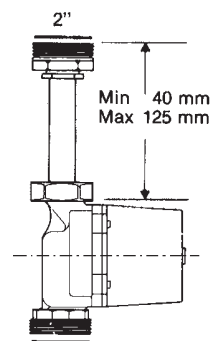
Переход с резьбы 1 1/2" на резьбу 2" с удлинителем
