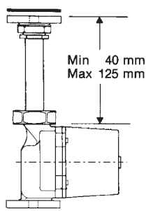
Переход с резьбового патрубка 1 1/2" на фланец DN25 - DN32, удлинитель с резьбой 1 1/2".
