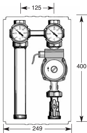
Насосный модуль NM (Без смесительного клапана)
