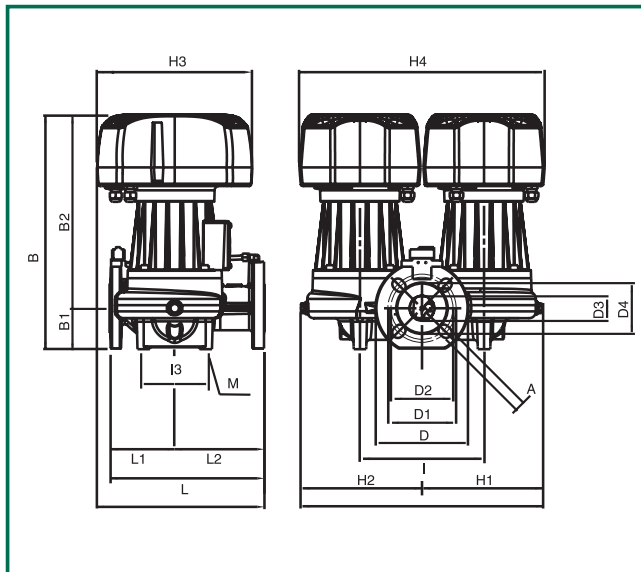
Габаритные размеры
