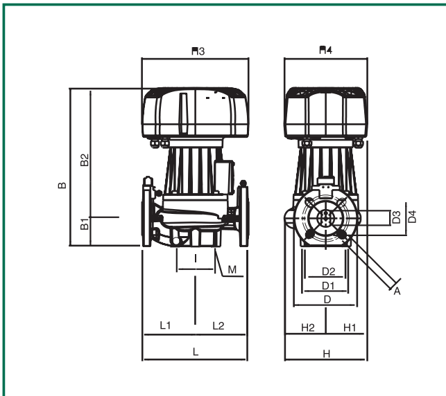
Габаритные размеры
