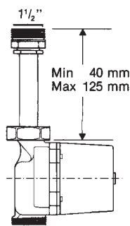
Удлинитель с резьбой 1 1/2"
