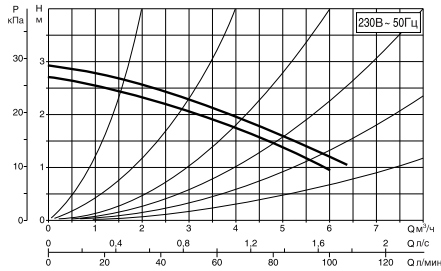
ВРН 60/250.40 Т
