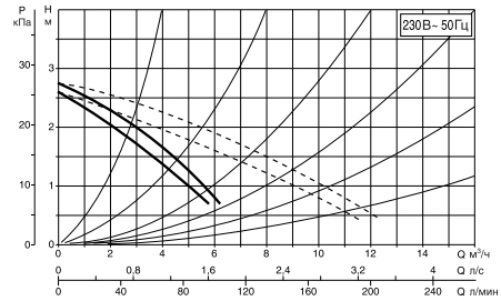
ДРН 60/250.40 Т
