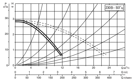
ДМН 60/280.50 Т
