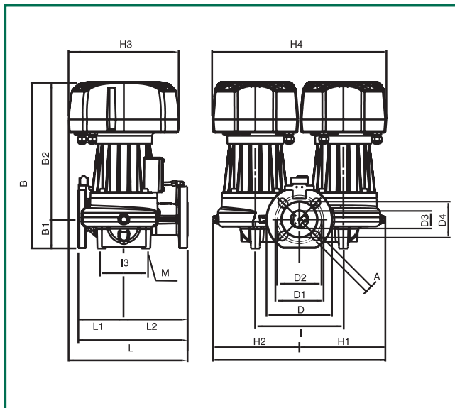
Габаритные размеры
