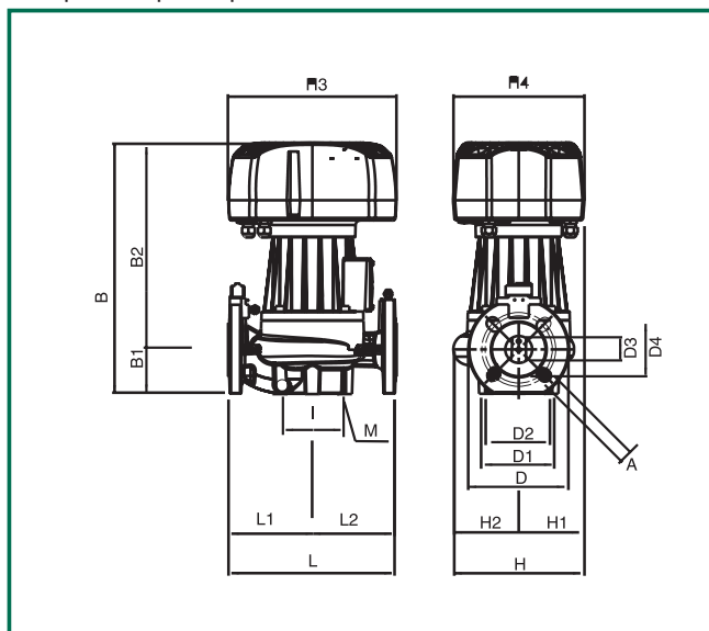
Габаритные размеры
