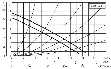
ВМН 30/280.50 Т
