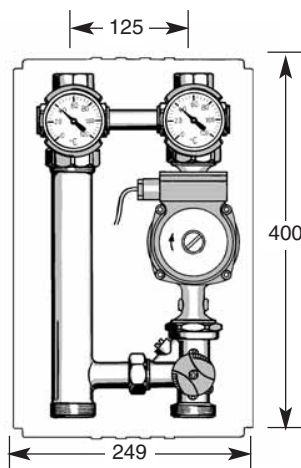
Насосный модуль M3 (Со смесительным клапаном)
