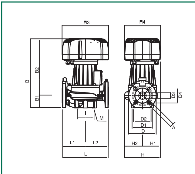
Габаритные размеры
