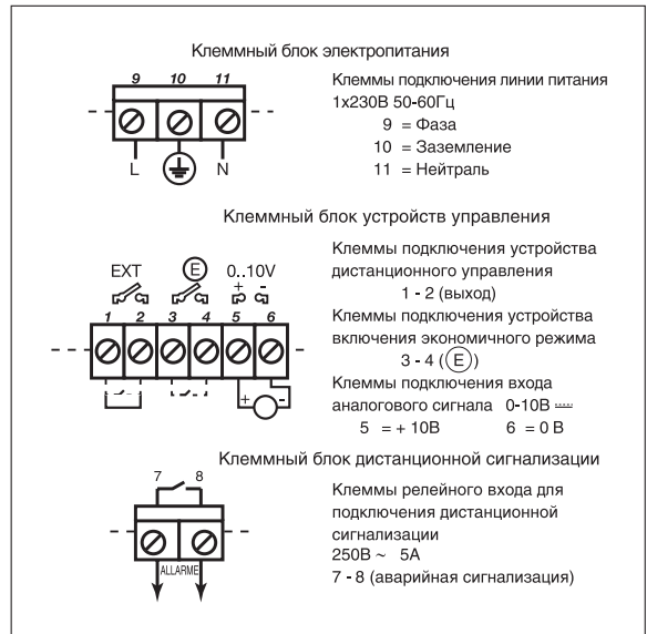
Клеммные соединения в электронном модуле
