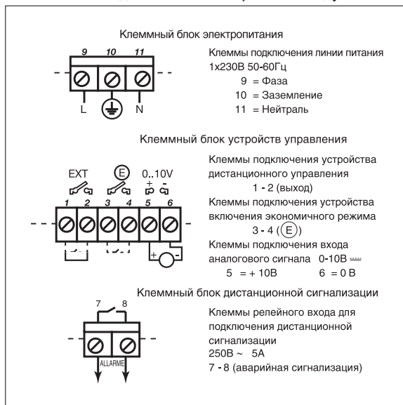
Клеммные соединения в электронном модуле
