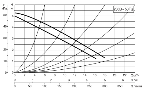
ВМН 60/280.50 Т
