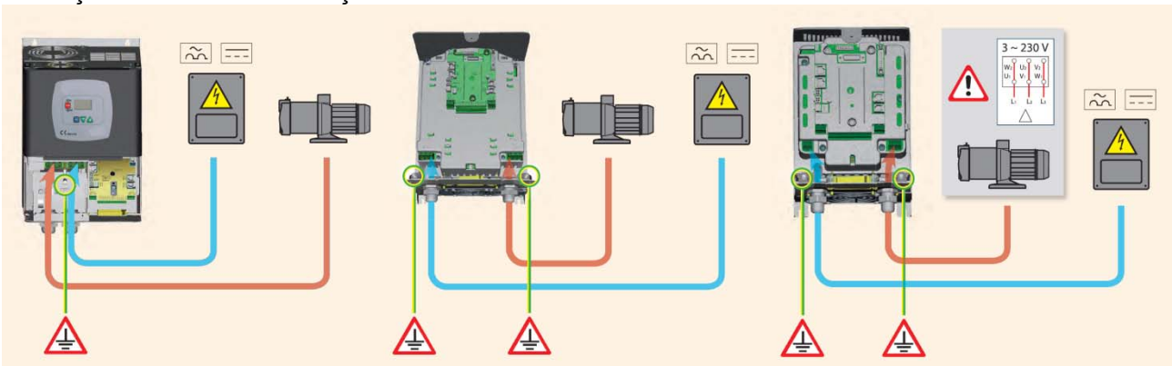
Figura 4: Conectări electrice
