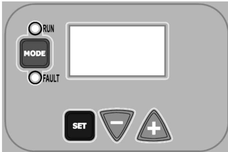
Fig. 12: Gränssnittets utseende
