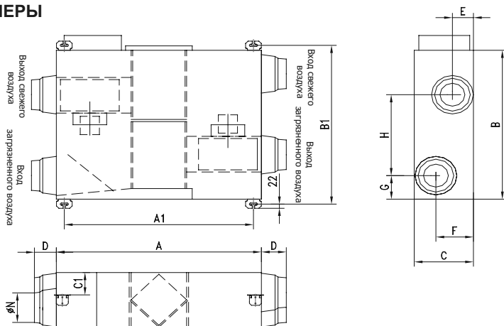
Рисунок 10 Размеры
