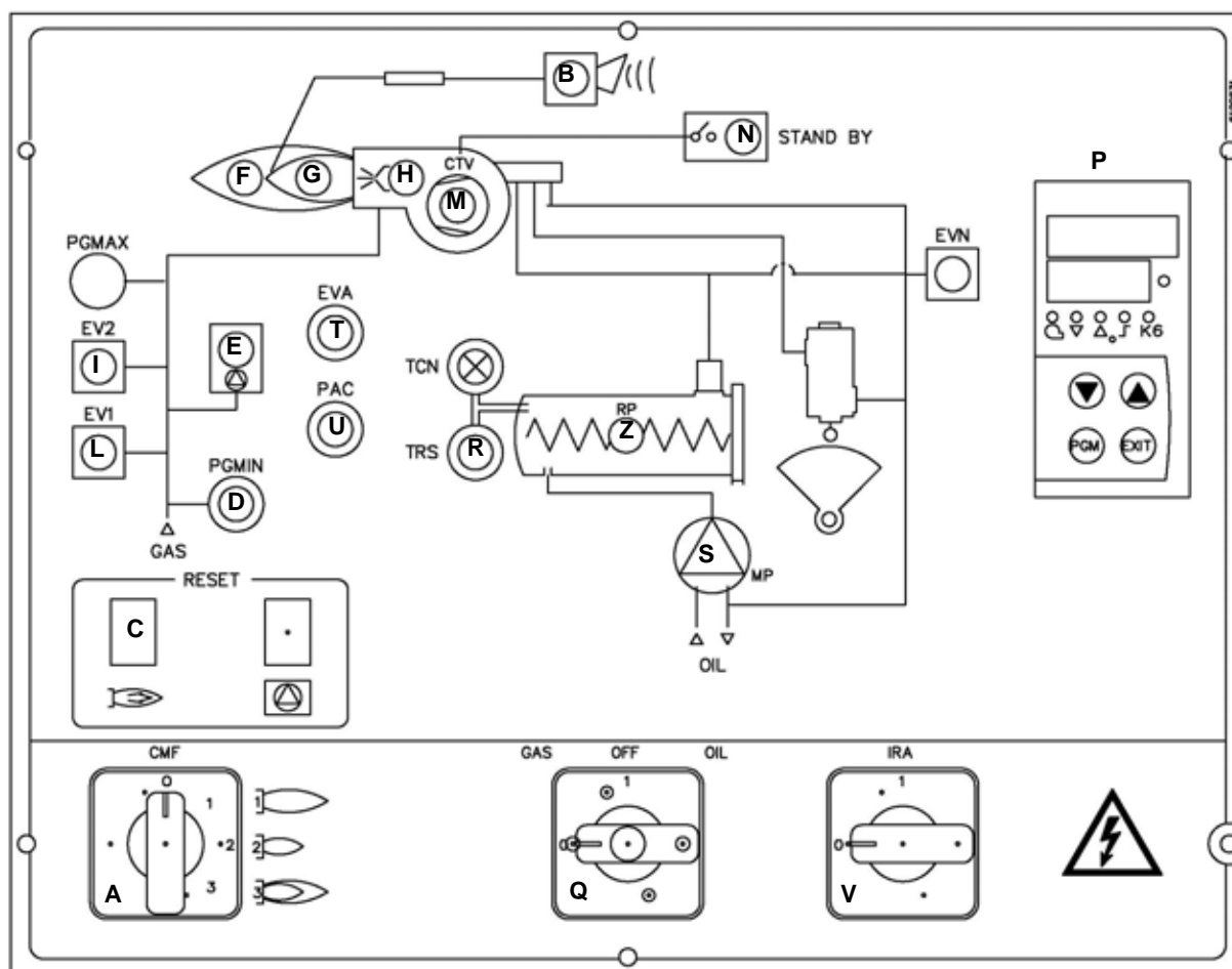
Рис. 24 - Передняя панель электрощита горелки
