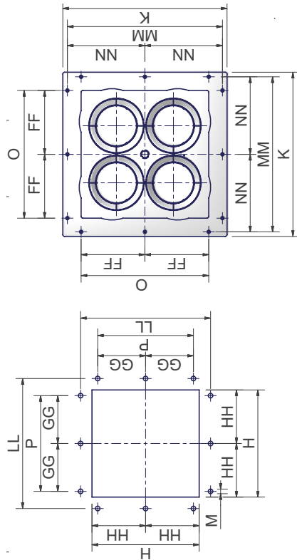
Рис. 2 - амбразура котла и фланцы горелок
