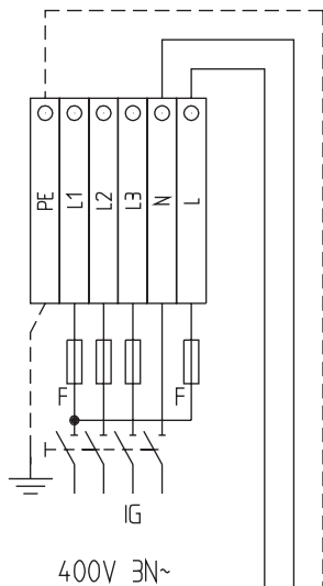
Электрощит QG - Клеммник МА1 Клеммник питания - пластина 1
