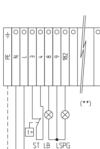
Электрощит QG - Клеммник МА2 Клеммник питания - пластина 2
