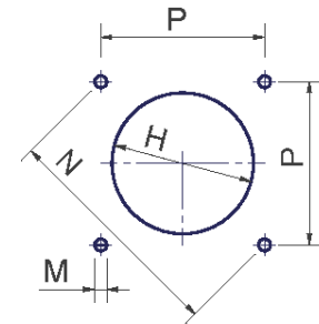
Рекомендуемая амбразура котла
