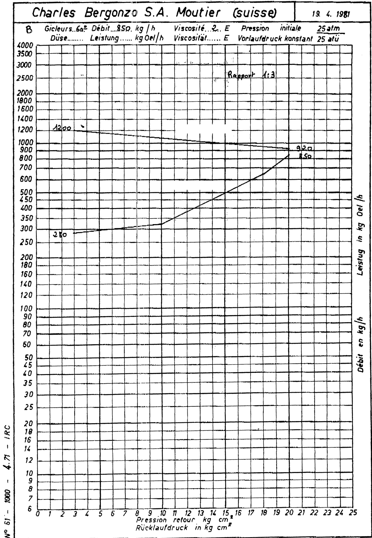
Рис. 20 - ФОРСУНКА BERGONZO - Пример с форсункой с расходом 850 кг/час
