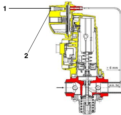
Исполнительный механизм "SKP"
