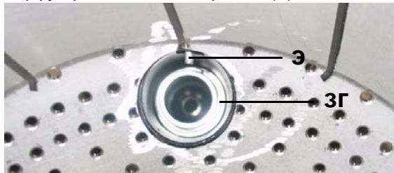
Рис. 27 - Часть диффузора с запальной горелкой (P) и запальным электродом (E).
