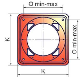
Фланец горелки
