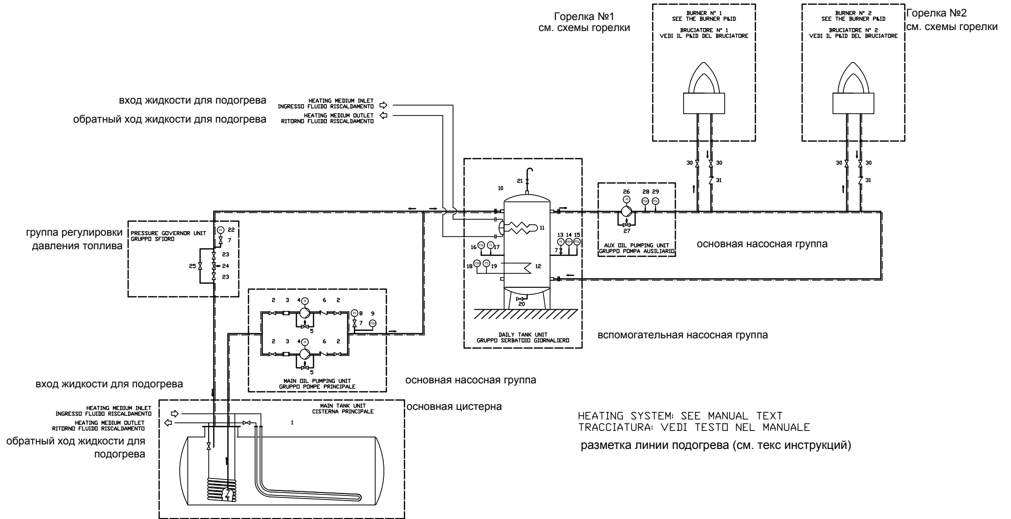
Рис. 30 - 31D0081 – Гидравлическая схема
