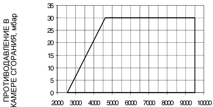
HR1030 DN65
