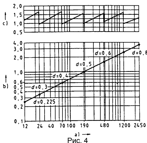
Рис. 4 - Тепловая нагрузка, диаметр и длина испытываемой топки, в зависимости от топочной мощности в кВт.
