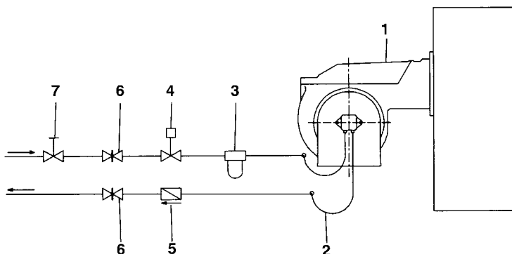
Fig. 7 - Двухтрубная система
