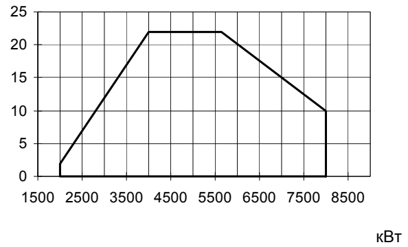
R525A M-....VS.1.50/65/80/100
