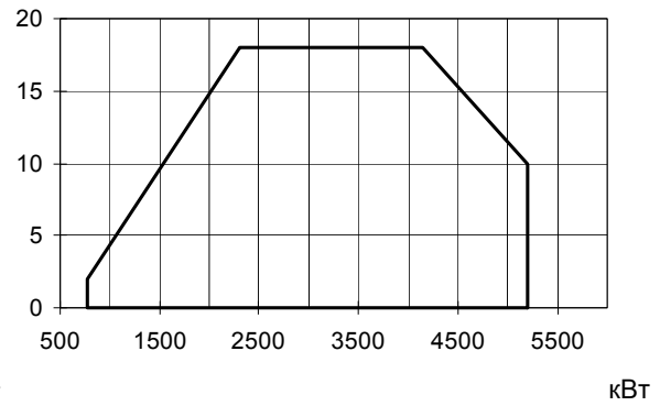
R515A M-....VS.1.50/65/80/100/
