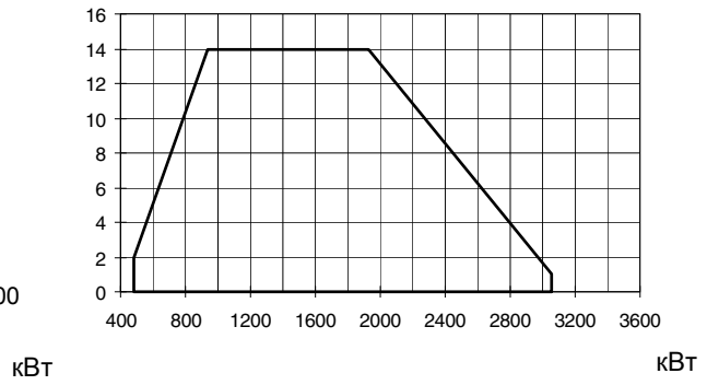
R515A M-....VS.1.50/65/80/100/
