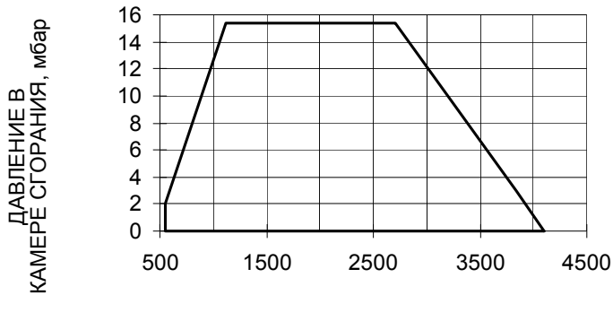
R520A M-....VS.x.50/65/80/100
