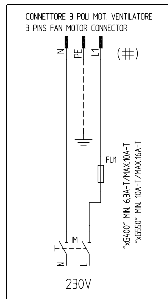
Рис. 39: 3-х полюсный соединительный разъем электродвигателя для NG/LG/NGX400
