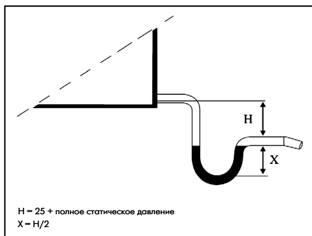
Рис. 8. Расчет дренажного сифона
