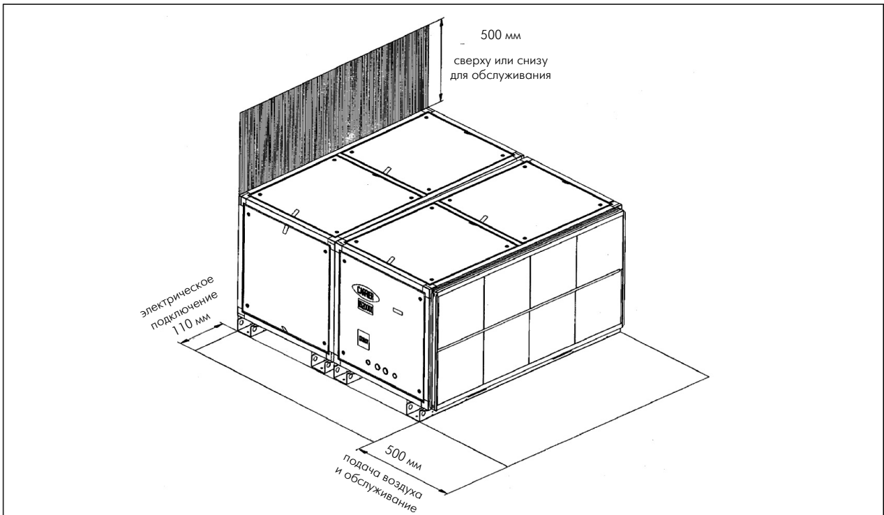
Рис. 3 - Минимальные зазоры вокруг агрегата
