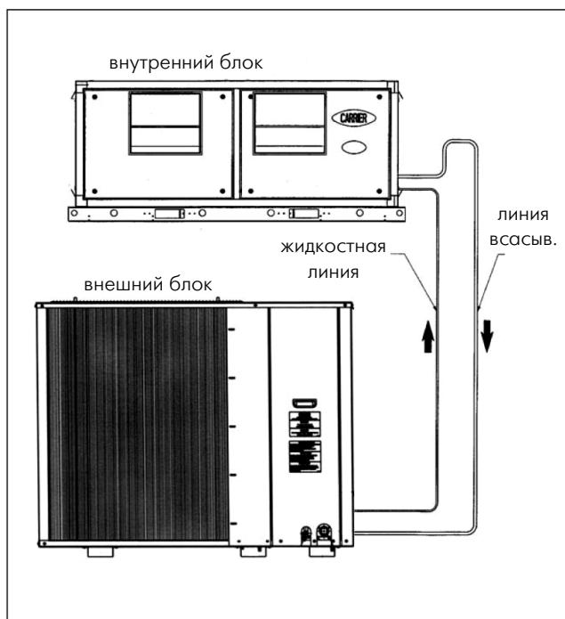
Рис. 6а. Конструкция трубопровода (внутренний блок выше внешнего)
