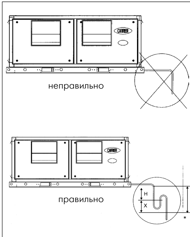
Рис. 7. Дренаж конденсата (* - общая высота сифона)
