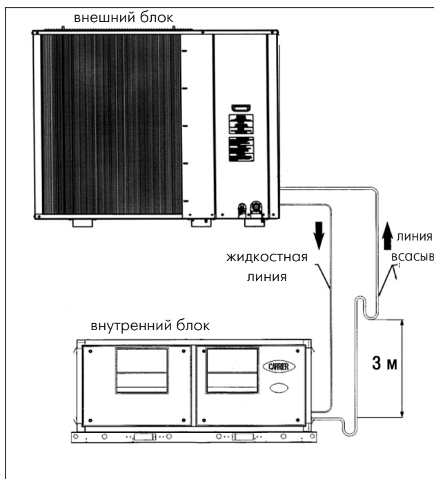
Рис. 6б. Конструкция трубопровода (внутренний блок ниже внешнего)
