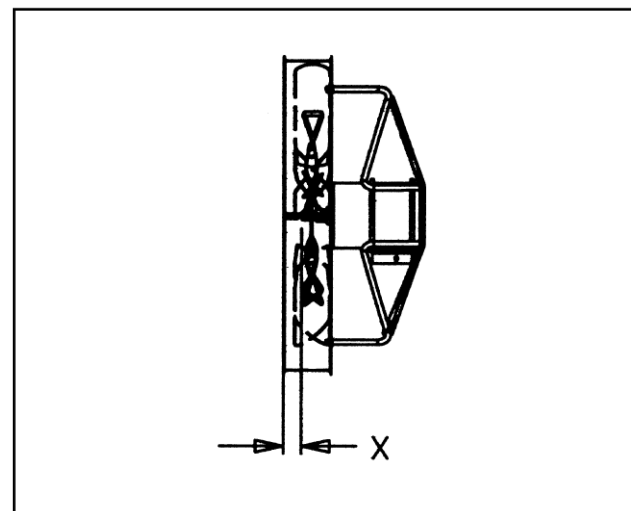
Рис. 10 Положение вентилятора
