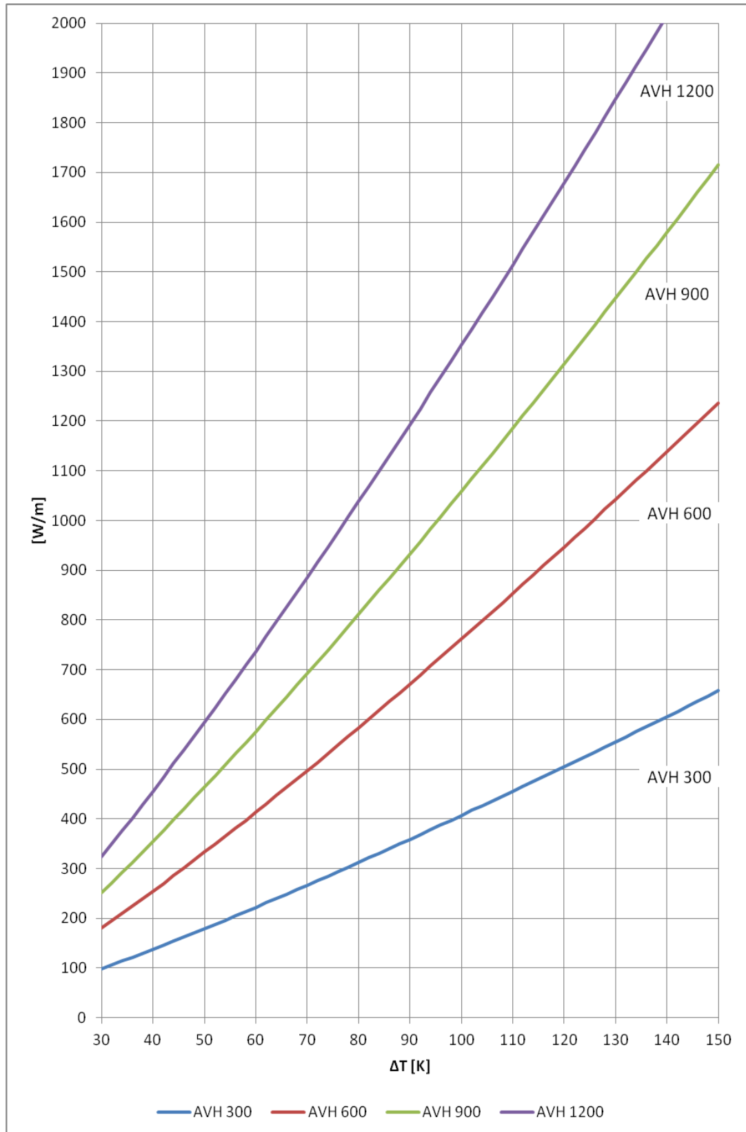
Рисунок 1.18 Тепловое излучение EUTERM AVH в соответствии с EN 14037-1 , -2, -3
