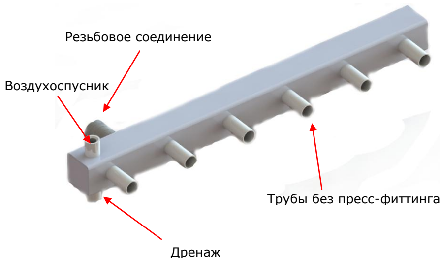
Рисунок 1.9 Компоненты коллектора
