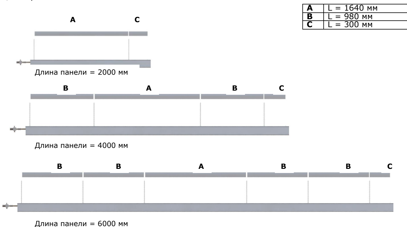
Рисунок 3.28 Позиции покрытия
