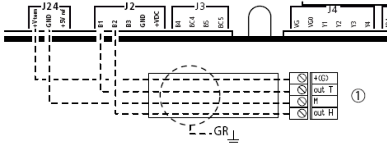
(1) Датчик температуры и датчик-ограничитель влажности
