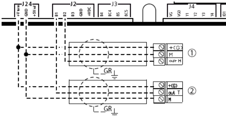
(1) Датчик-ограничитель влажности
