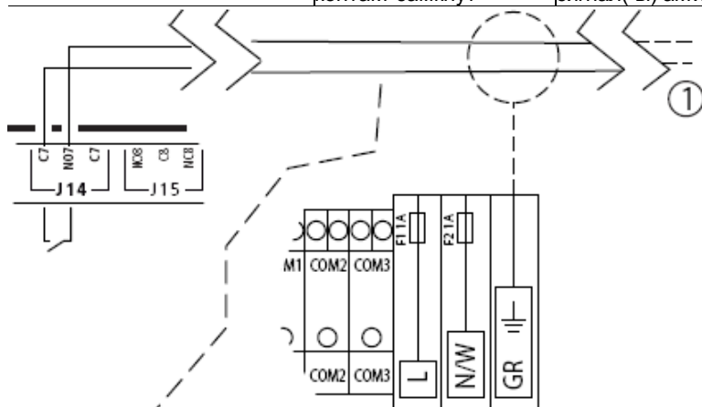
(1) Реле сигналов неисправности
