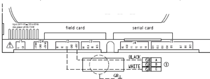
(1) Датчик давления
