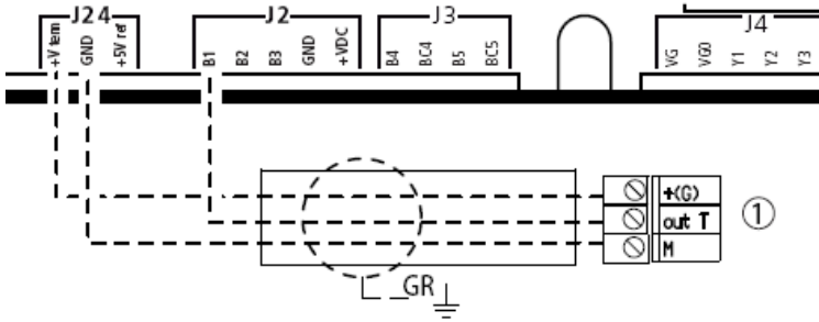
(1) Датчик температуры
