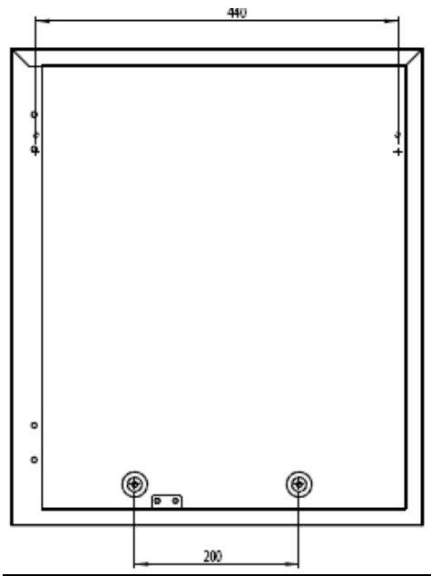
Тыльная сторона шкафа управления
