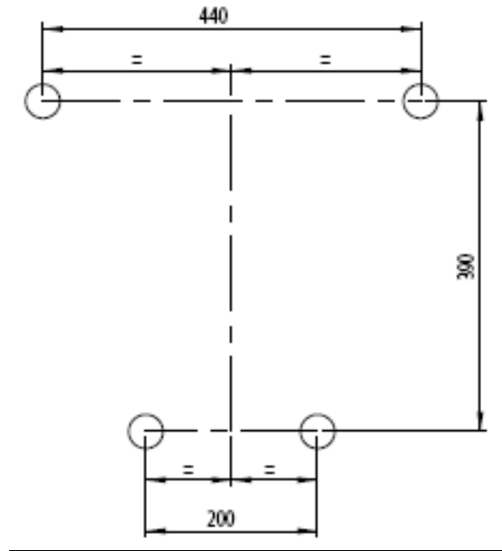
Шаблон для сверления
