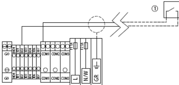
(1) гигростат ВКЛ/ВЫКЛ
