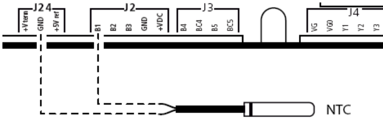
(1) Датчик NTC
