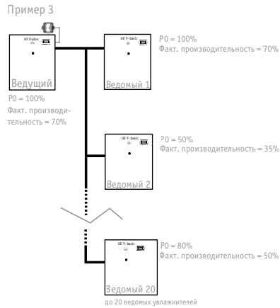
Схема соединения ведущего UEX и ведомых UEY с помощью экранированных проводов
