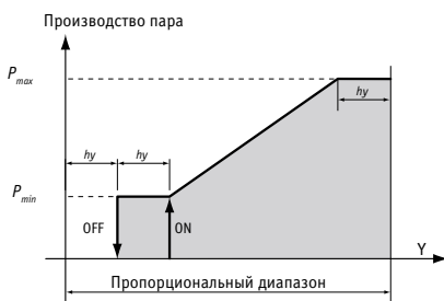
Рис. 14.а Пропорциональное управление
