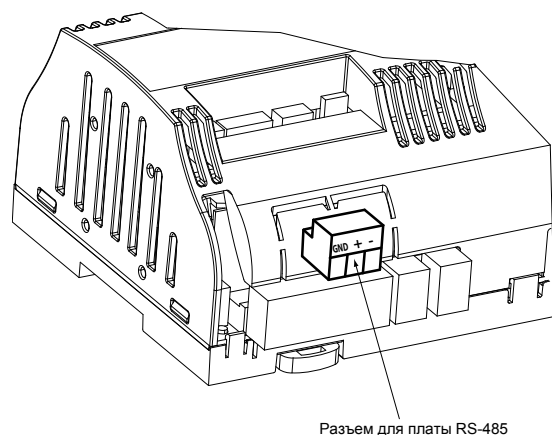
Разъем для платы RS-485
