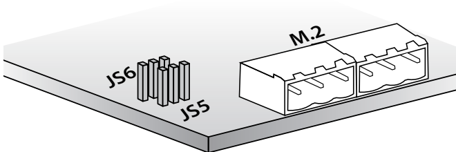
Рис. 4.м (деталь электронной платы в электрической секции увлажнителя)
