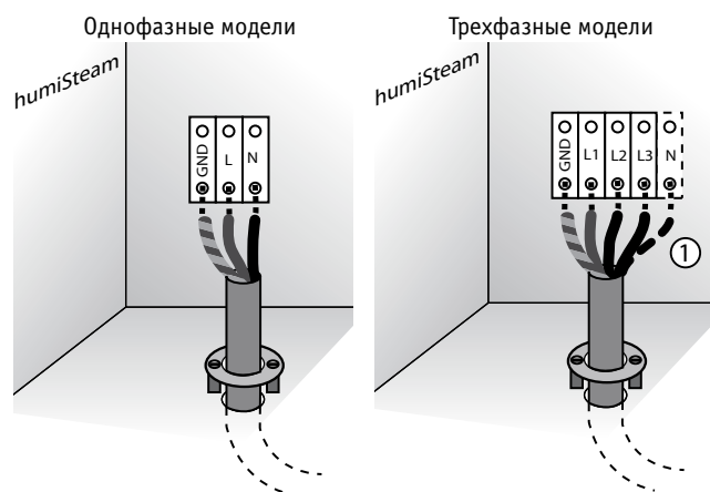
Рис. 4.с (вид внутри агрегата, электрическая секция)
