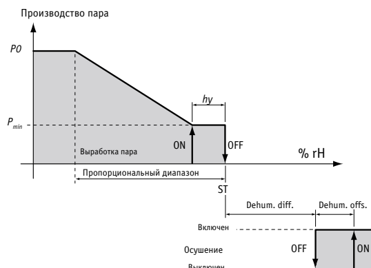
Рис. 14.б Управление от датчика влажности
