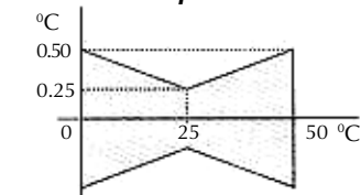
Измерение температуры (резистивный NTC-датчик) в диапазоне 0-50 °C
