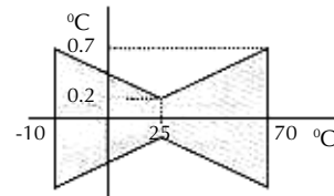
Измерение температуры (датчик Pt1000) в диапазоне -10-70 °C
