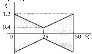
Измерение температуры (активный NTC-датчик) в диапазоне 0-50 °C
