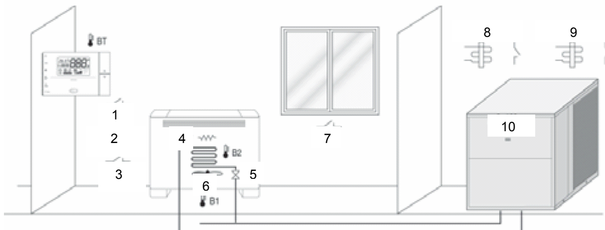
Пример установки фэн-койла в 2-трубной системе Рис. 4.а.
