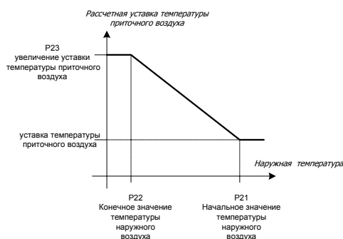
Зимняя компенсация уставки температуры приточного воздуха по наружной температуры
