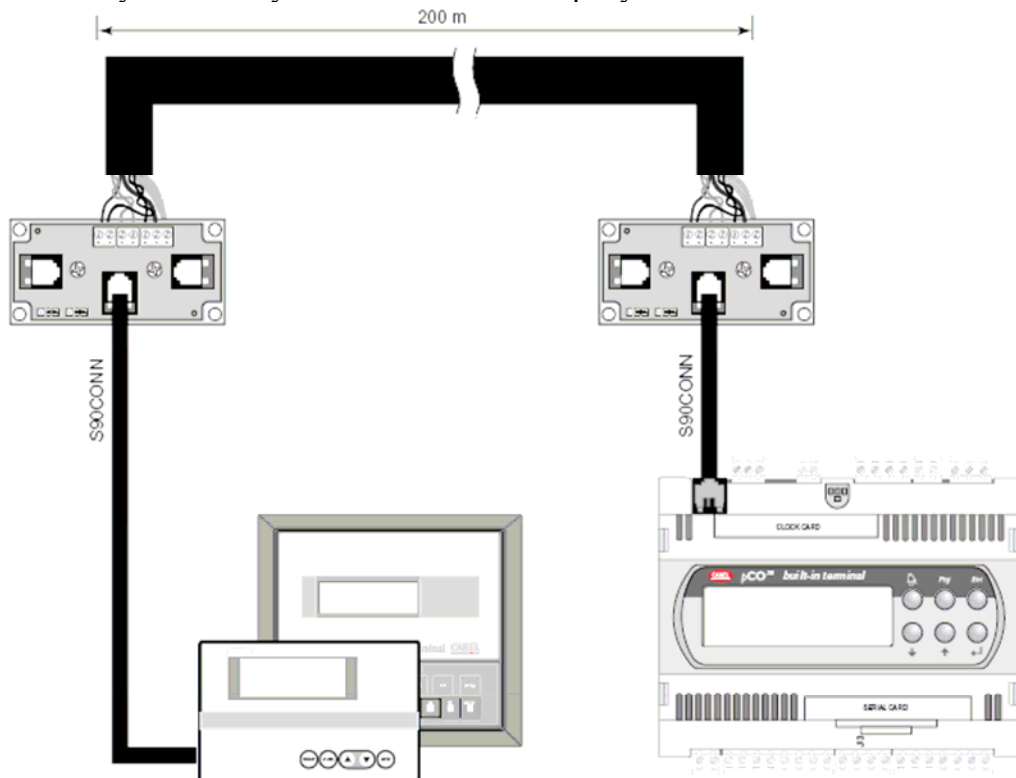
Рисунок 5.5.2.2 пердстает шунт TCONN6J000 , используемый в паре для удаленной установки pCOxs в сети pLAN с экранированным кабелем AWG24
