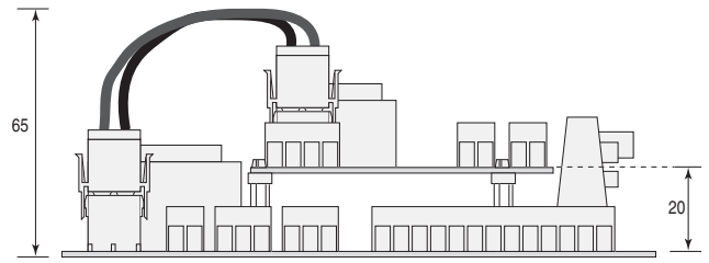
Fig. 3.10: altezza e-drofan con accessori / e-drofan high accessories included
